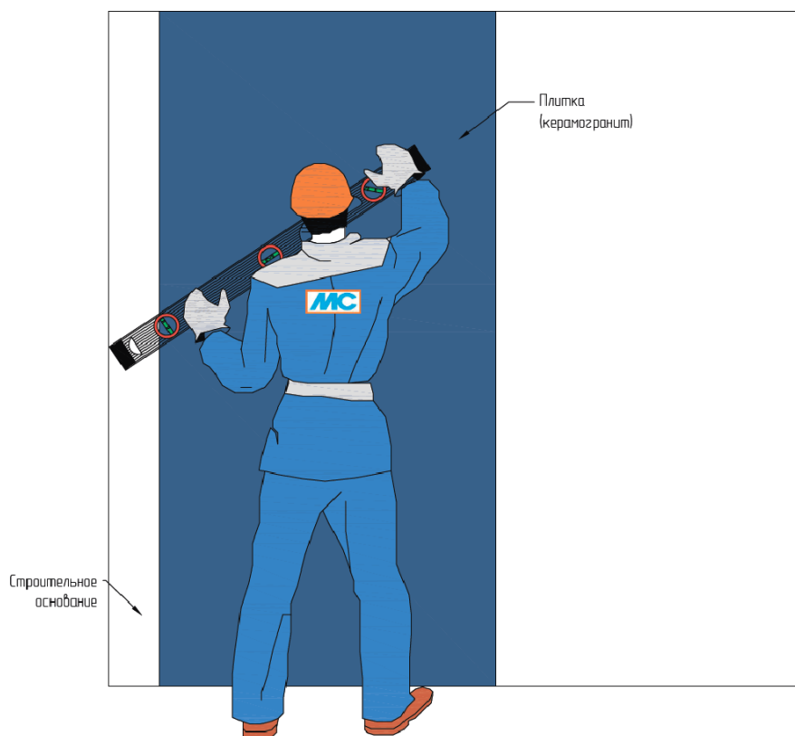
Рис. 18. Проверка облицовки при помощи уровня
