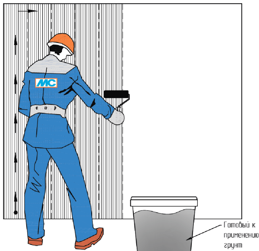
Рис. 10. Схема организации работ по нанесению грунта на основание
