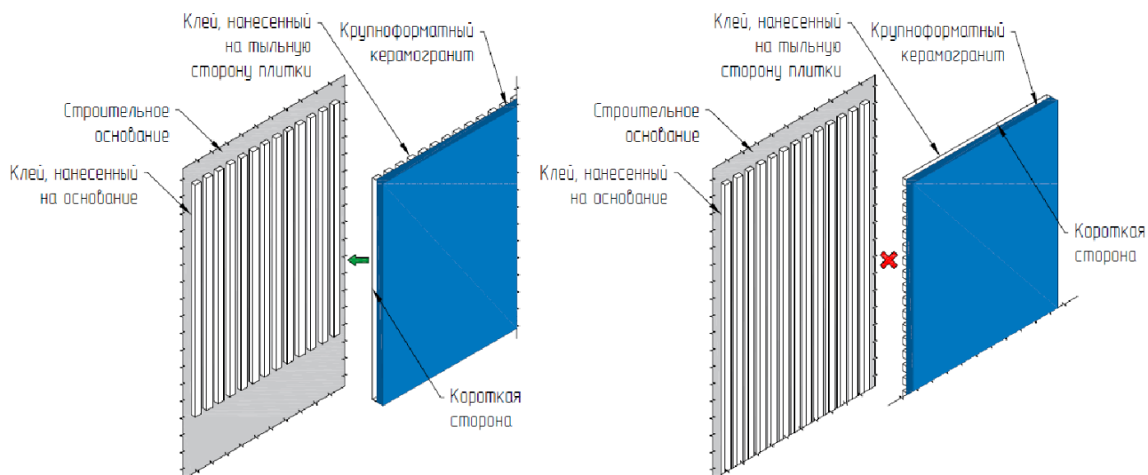
Рис. 12. Клей следует наносить в одном направлении на основание и на плитку
