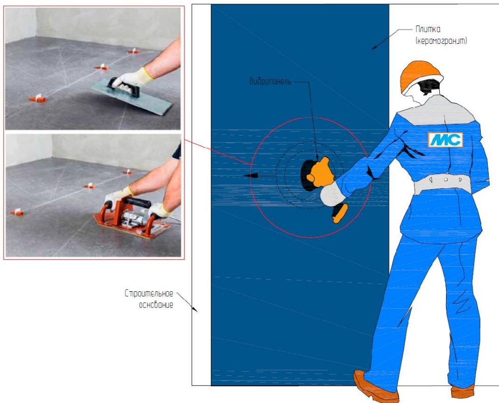
Рис. 17. Увеличение адгезии плитки с основанием вибрированием или простукиванием
