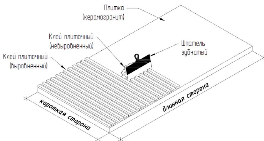
Рис. 11. Нанесение плиточного клея на плитку
