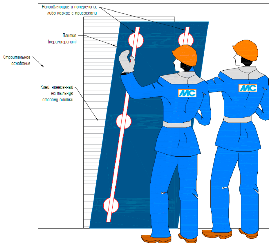
Рис. 16. Монтаж крупноформатного керамогранита
