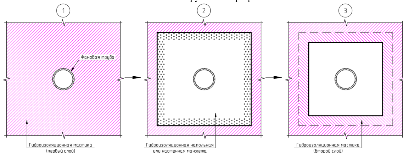
Рис.30.4. Последовательность нанесения гидроизоляционной манжеты.
