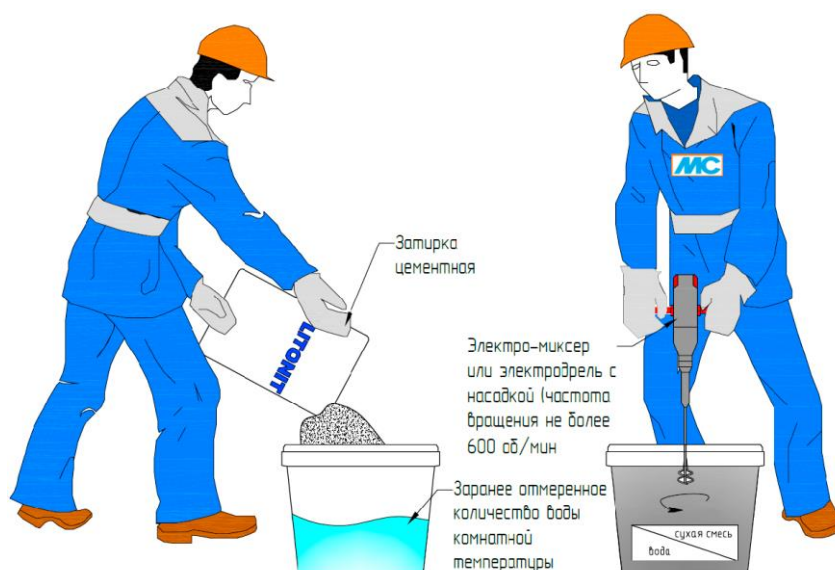
Рис. 35. Приготовление состава
