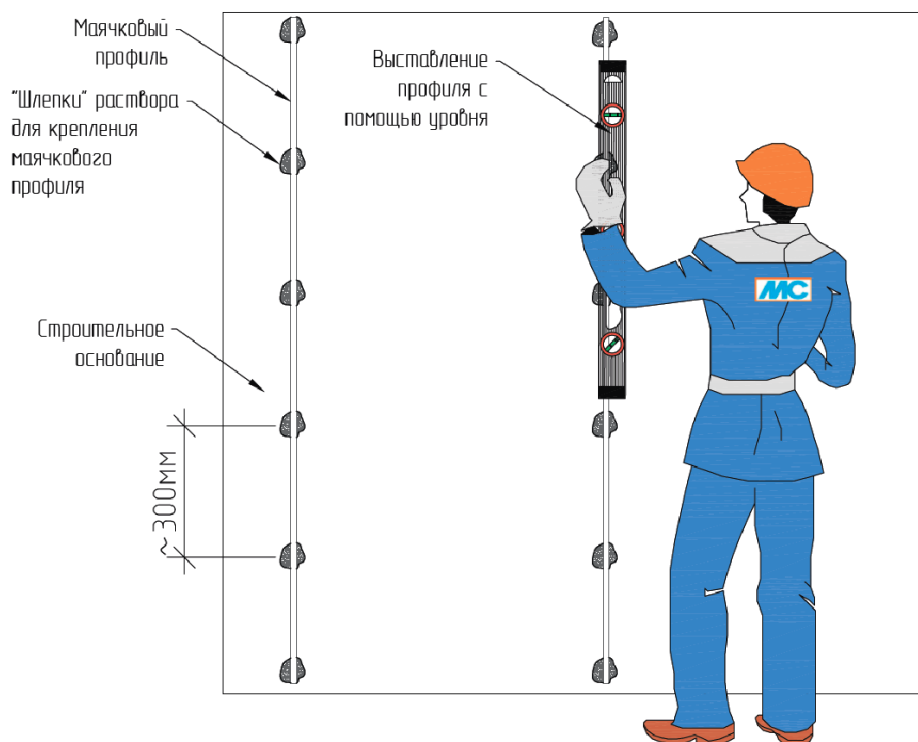
Рис.19. Монтаж маяка с помощью правила с уровнем
