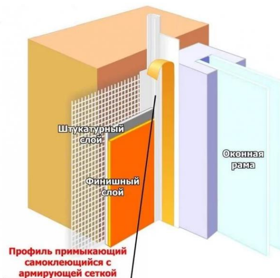
Рис.22. Профиль примыкающий с армирующей сеткой
