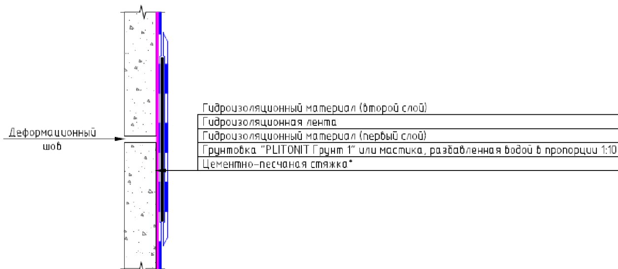
Рис.30.3. Конструктивный разрез №3.
