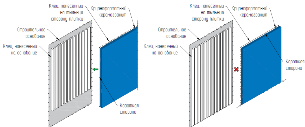
Рис. 21. Клей следует наносить в одном направлении на основание и на плитку
