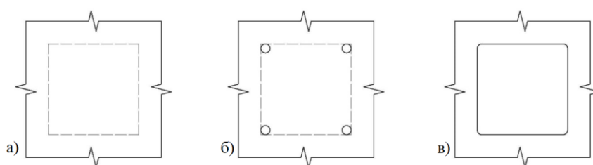
Рис. 24. Резка прямоугольных отверстий
