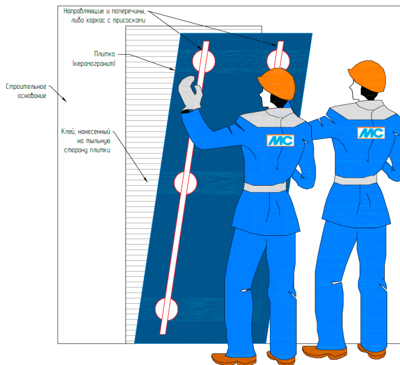
Рис. 25. Монтаж крупноформатного керамогранита
