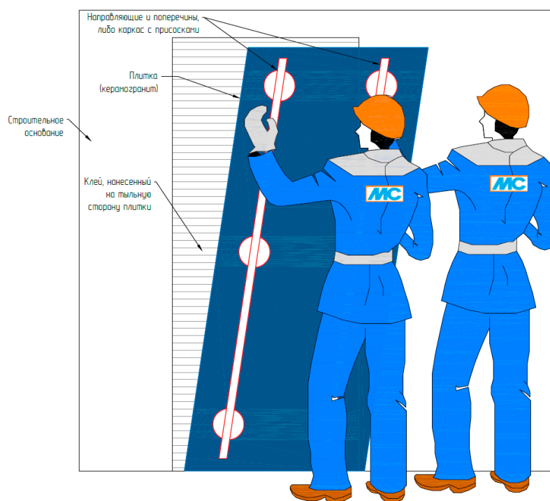
Рис. 30. Монтаж крупноформатного керамогранита
