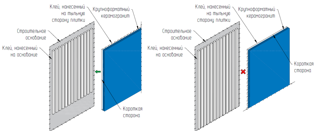
Рис. 26. Клей следует наносить в одном направлении на основание и на плитку
