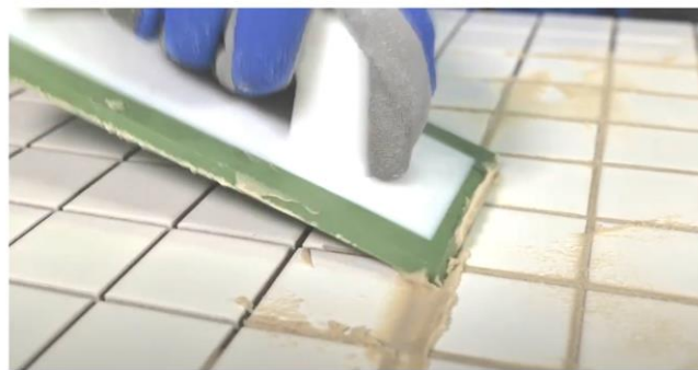
Рис. 25. Заполнение швов затиркой при помощи резинового шпателя
