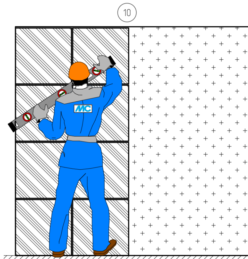
Рис.22. Последовательность работ, где: 1 – проверка ровности основания контрольной рейкой; 2, 3 – приготовление грунтовки; 4 – нанесение грунтовки на цементную штукатурку; 5 – приготовление клеевой смеси; 6, 7 – нанесение клеевой смеси на основание (захватками); 8, 9 – приклеивание керамогранитной плитки на стену (захватками); 10 – проверка облицовки при помощи уровня.
