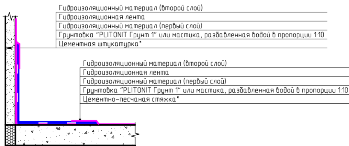
Разрез 1-1
