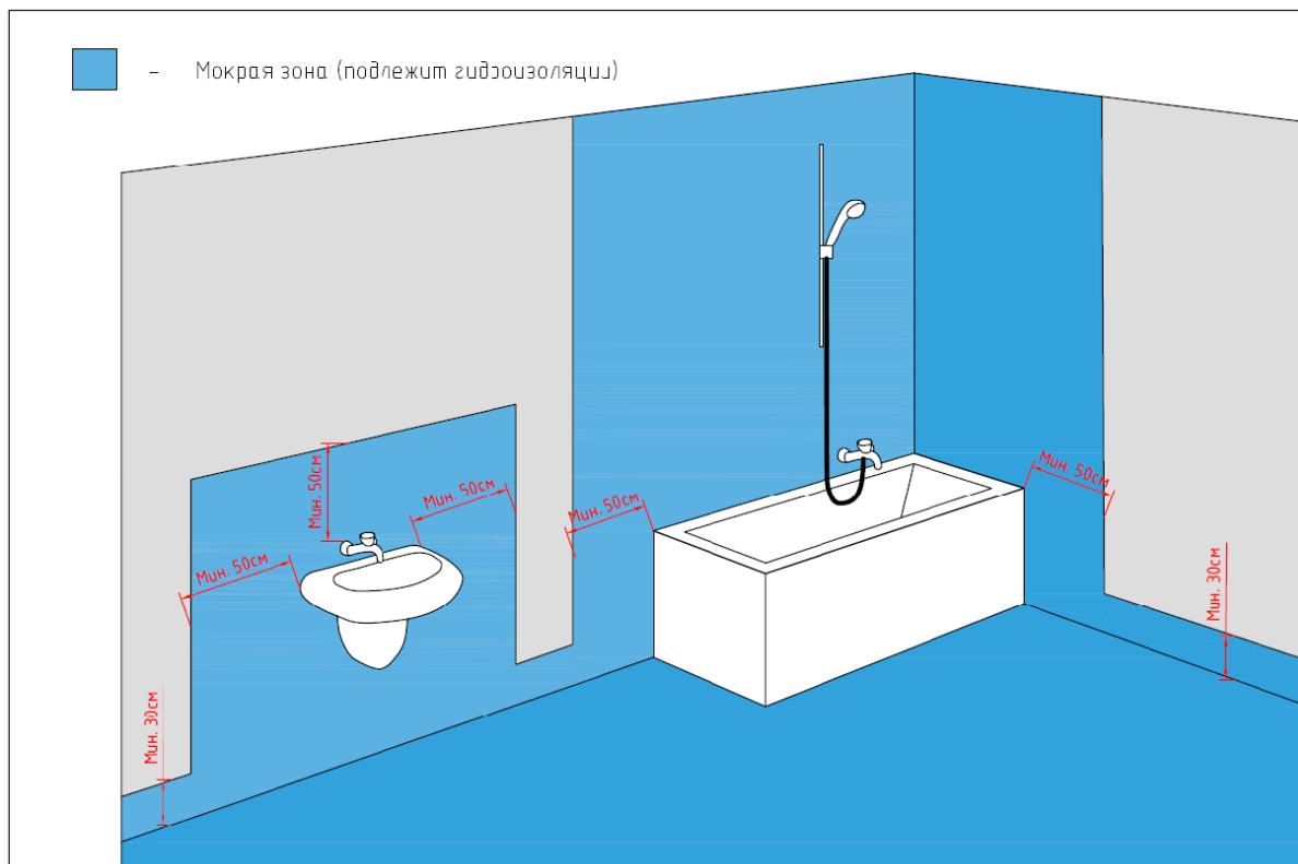
Рис. 13.2 Мокрые зоны внутри влажных помещений, подлежащие гидроизоляции.
