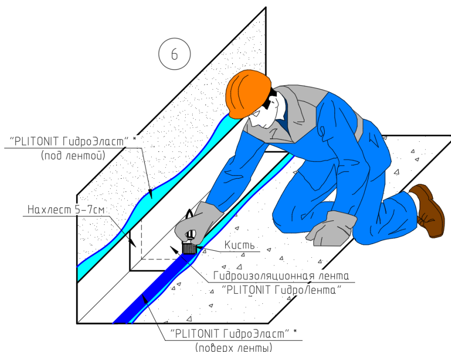
Рис.13.1. Последовательность работ (на стенах работа в аналогичном порядке), где: 1 - проверка ровности основания контрольной рейкой (аналогично для горизонтальной поверхности); 2 – размешивание емкости с мастикой; 3 – нанесение первого слоя мастики, разбавленной водой в пропорции 1:10, на основание; 4 – нанесение гидроизоляции на поверхность (аналогично для горизонтальной поверхности); 5 – укладка гидроизоляционной ленты на поверхность, предварительно обработанную «PLITONIT ГидроЭласт» или «PLITONIT WaterProof Standard»; 6 – поверхностная обработка ленты мастикой «PLITONIT ГидроЭласт» или «PLITONIT WaterProof Standard».
