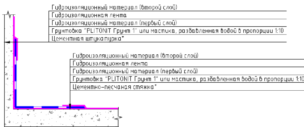
Разрез 1-1
