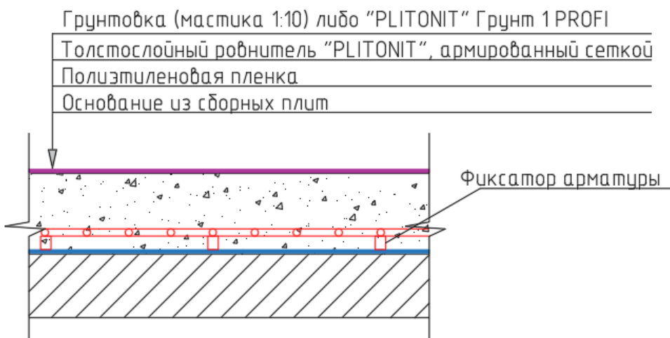
Рис.18. Конструктивный разрез №2.
