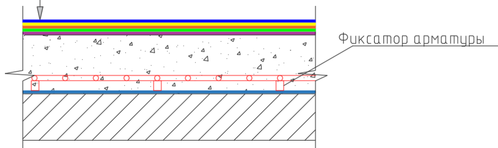
Рис.21. Конструктивный разрез №5.
