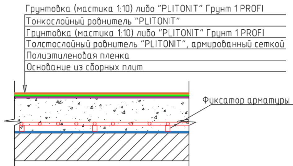
Рис.20. Конструктивный разрез №4.
