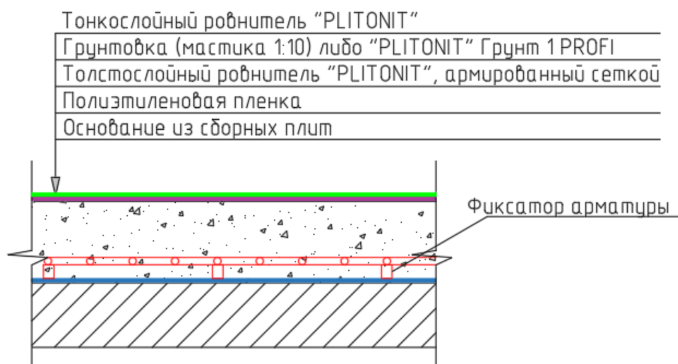
Рис.19. Конструктивный разрез №3.
