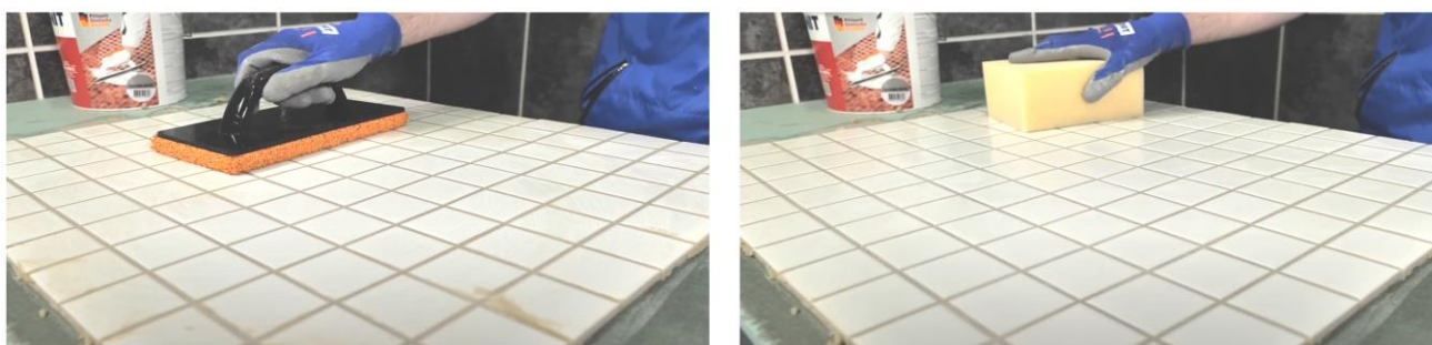
Рис. 25. Диагональными движениями шпателя убрать с поверхности плитки излишки затирки
