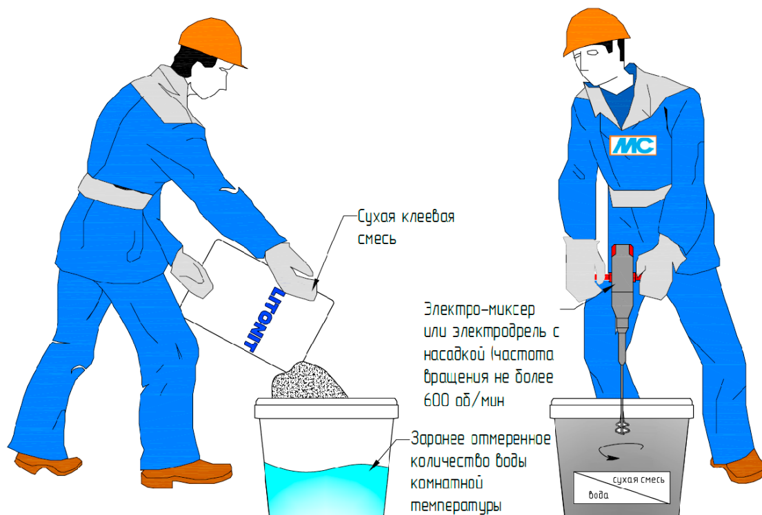
Рис. 19. Организация работ по затворению сухой клеевой смеси
