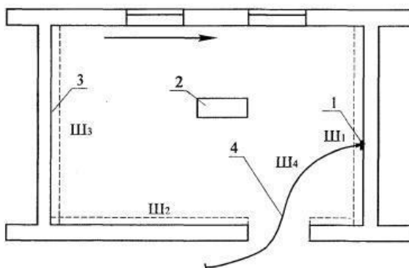
Рис.15. Схема организации рабочего места звена № 1
