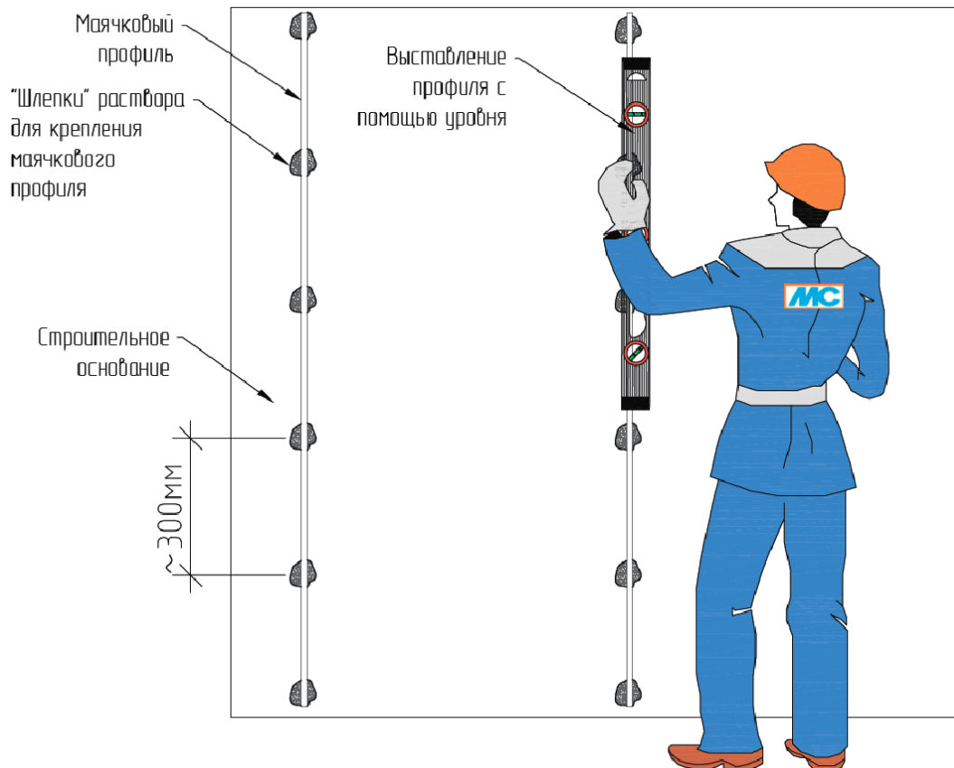
Рис.11. Монтаж маяка с помощью правила с уровнем
