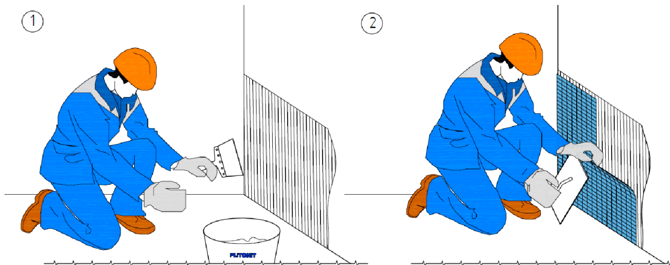
Рис. 20. Организация работ по приклеиванию мозаики
