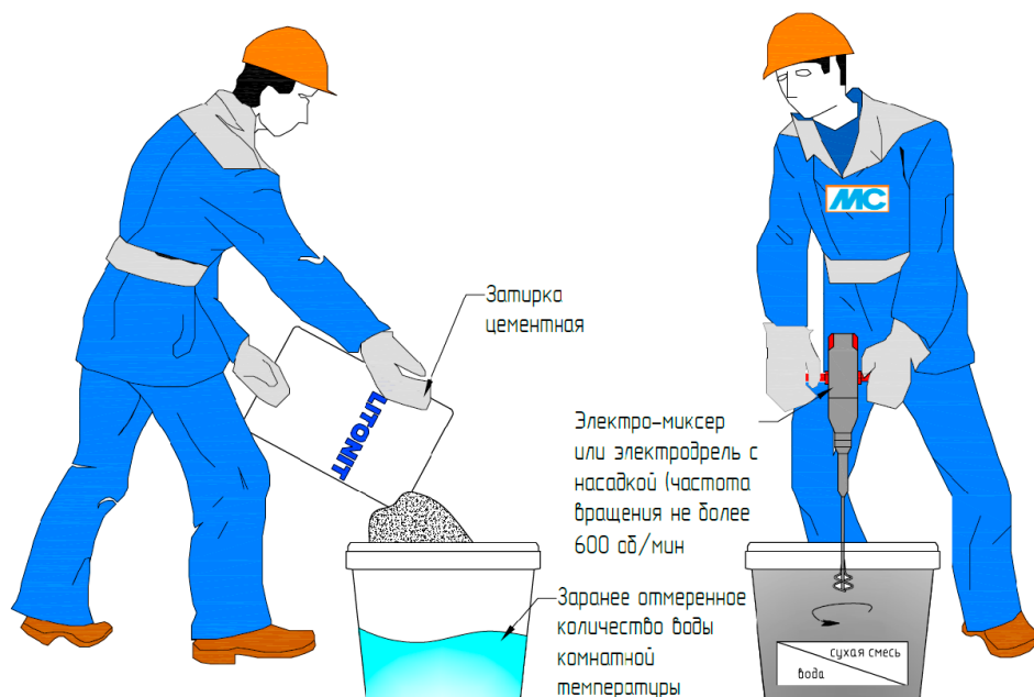
Рис. 22. Приготовление состава
