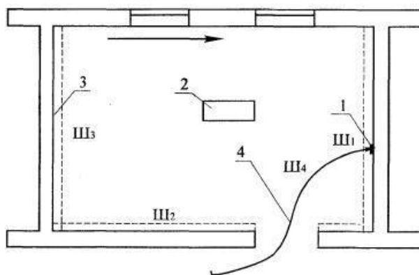
Рис. 23. Схема организации рабочего места звена № 1
