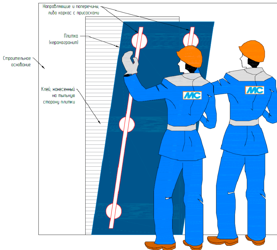
Рис. 34. Монтаж крупноформатного керамогранита
