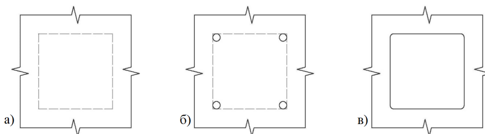
Рис. 33. Резка прямоугольных отверстий
