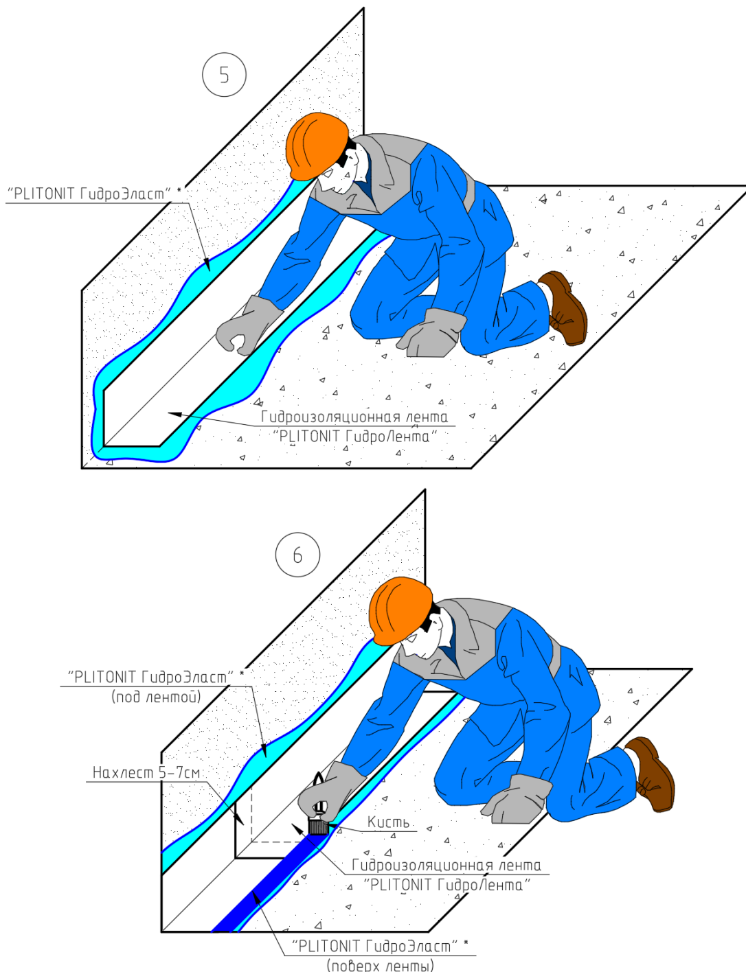
Рис.28. Последовательность работ, где: 1 - проверка ровности основания контрольной рейкой (аналогично для горизонтальной поверхности); 2 – размешивание емкости с мастикой; 3 – нанесение первого слоя мастики, разбавленной водой в пропорции 1:10, на основание; 4 – нанесение гидроизоляции на поверхность (аналогично для горизонтальной поверхности); 5 – укладка гидроизоляционной ленты на поверхность, предварительно обработанную «PLITONIT ГидроЭласт» или «PLITONIT WaterProof Standard»; 6 – поверхностная обработка ленты мастикой «PLITONIT ГидроЭласт» или «PLITONIT WaterProof Standard».
