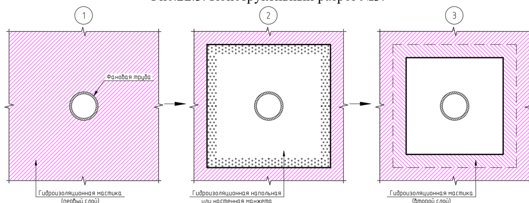
Рис.22.3. Конструктивный разрез №3.
