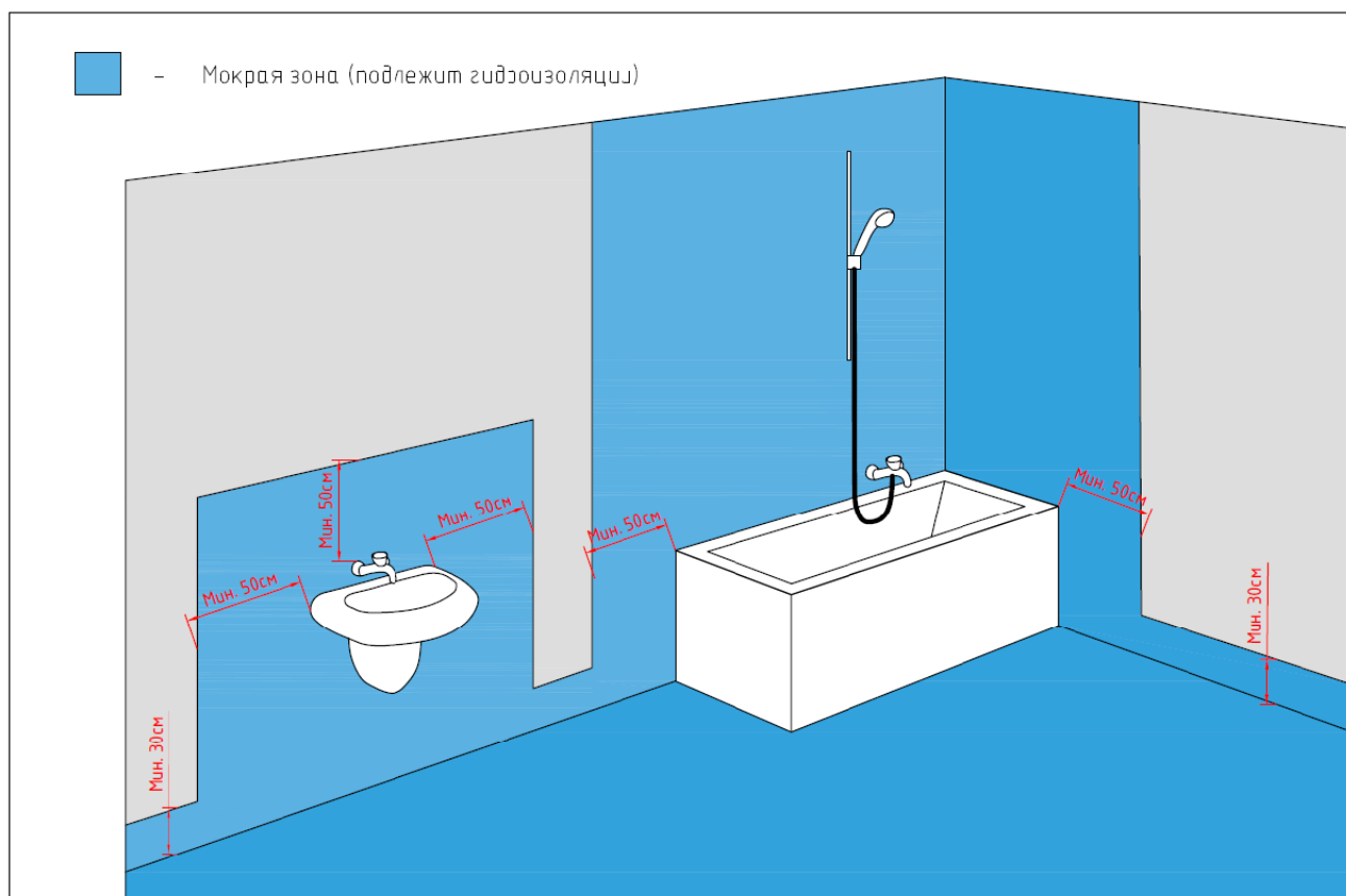
Рис. 23.2 Мокрые зоны внутри влажных помещений, подлежащие гидроизоляции.
