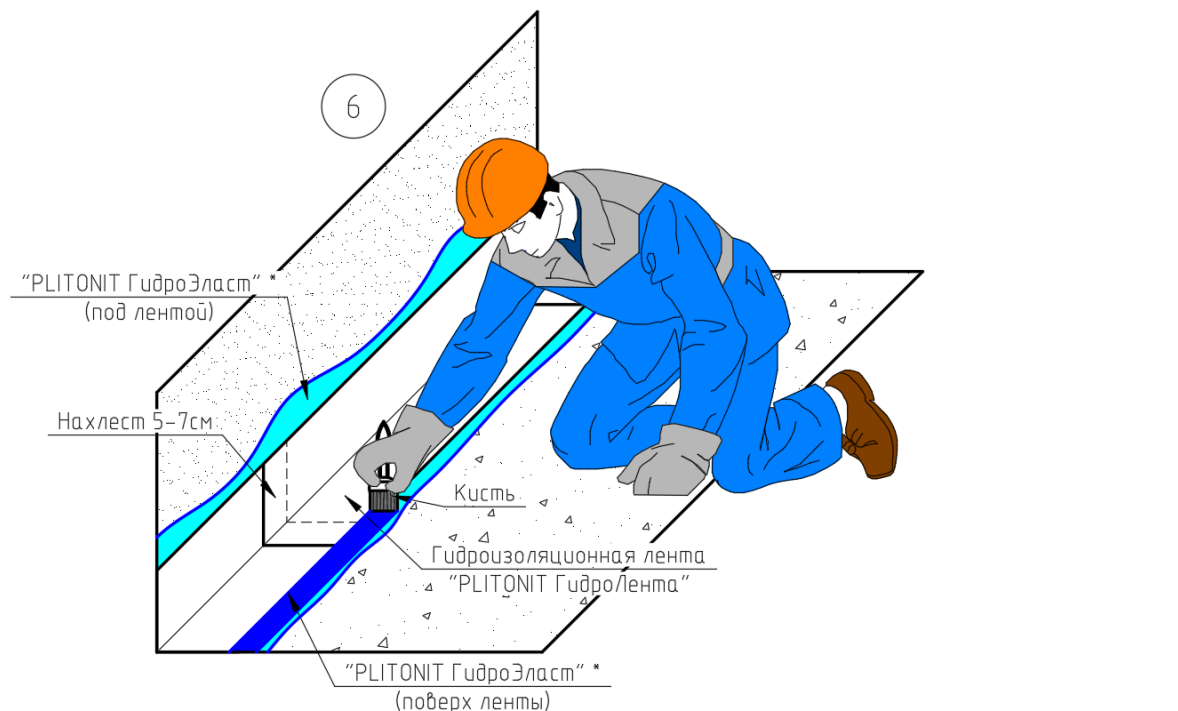
Рис.23.1. Последовательность работ (на стенах работа в аналогичном порядке), где: 1 - проверка ровности основания контрольной рейкой (аналогично для горизонтальной поверхности); 2 - размешивание емкости с мастикой; 3 - нанесение первого слоя мастики, разбавленной водой в пропорции 1:10, на основание; 4 - нанесение гидроизоляции на поверхность (аналогично для горизонтальной поверхности); 5 - укладка гидроизоляционной ленты на поверхность, предварительно обработанную «PLITONIT ГидроЭласт» или «PLITONIT WaterProof Standard»; 6 - поверхностная обработка ленты мастикой «PLITONIT ГидроЭласт» или «PLITONIT WaterProof Standard».
