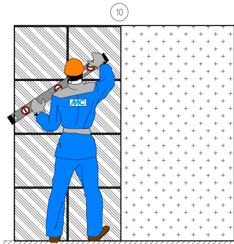
Рис.15. Последовательность работ, где: 1 – проверка ровности основания контрольной рейкой; 2, 3 – приготовление грунтовки; 4 – нанесение грунтовки на цементную штукатурку; 5 – приготовление клеевой смеси; 6, 7 – нанесение клеевой смеси на основание (захватками); 8, 9 – приклеивание керамогранитной плитки на стену (захватками); 10 – проверка облицовки при помощи уровня. ПРИМЕЧАНИЕ к рис 18.: на этапах 6-9 указано проведение работ в направлении снизу вверх, но при использовании клеев, в маркировке которых присутствует буква «Т», возможно выполнение работ в направлении сверху вниз.
