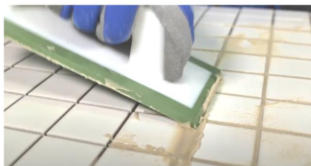
Рис. 29. Заполнение швов затиркой при помощи резинового шпателя
