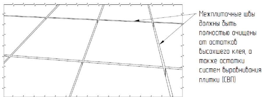
Рис. 27. Подготовка межплиточных швов
