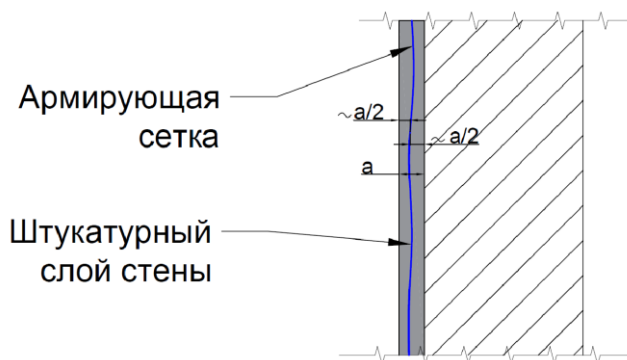
Рис. 25. Армированный штукатурный слой в местах стыка разных материалов стен
