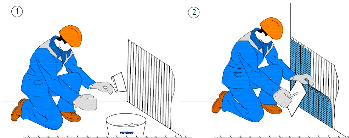
Рис. 33. Организация работ по приклеиванию мозаики
