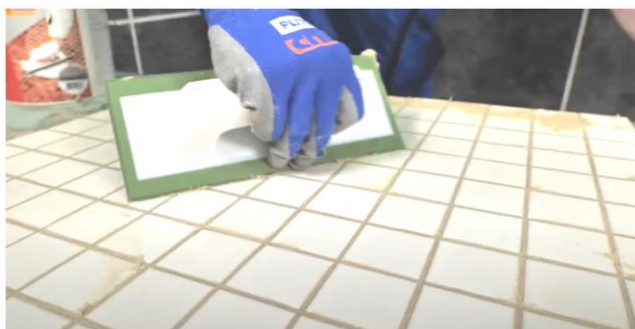
Рис. 37. Диагональными движениями шпателя убрать с поверхности плитки излишки затирки
