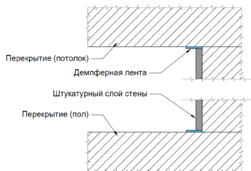
Рис.21. Приклейка демпферной ленты в местах сопряжения штукатурного слоя со стеной и потолком
