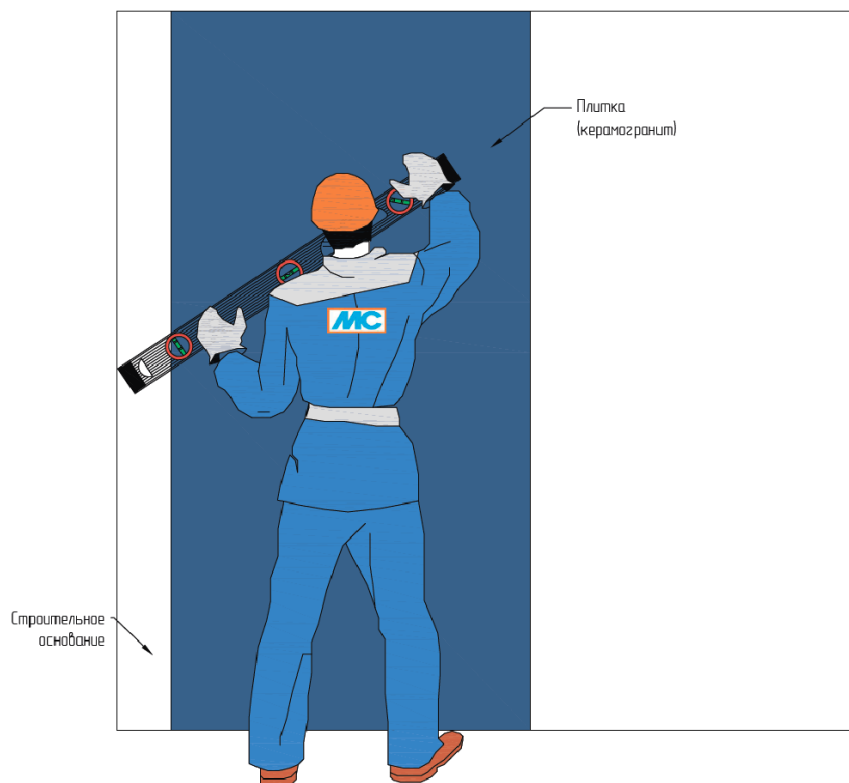
Рис. 37. Проверка облицовки при помощи уровня
