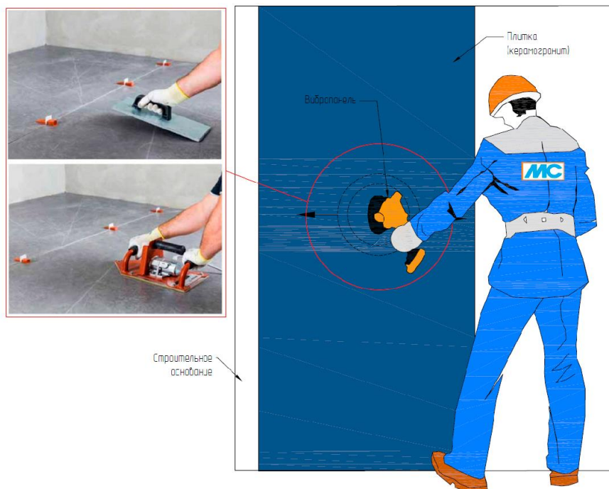
Рис. 36. Увеличение адгезии плитки с основанием вибрированием или простукиванием
