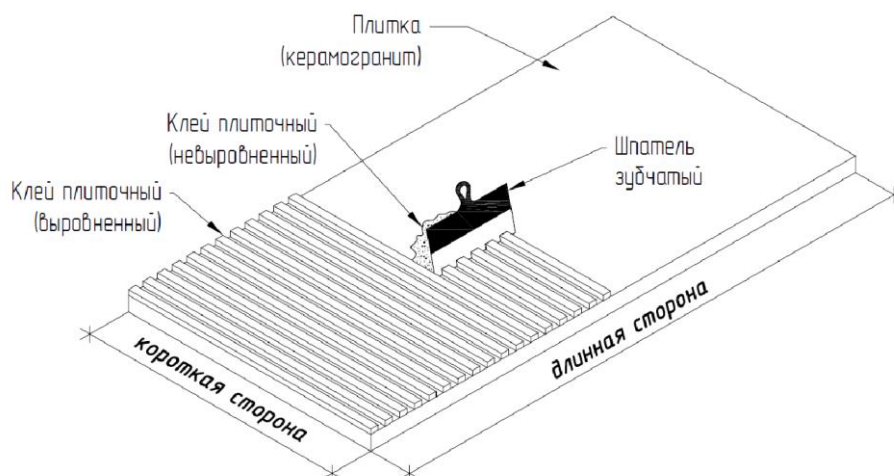
Рис. 31. Нанесение плиточного клея на плитку
