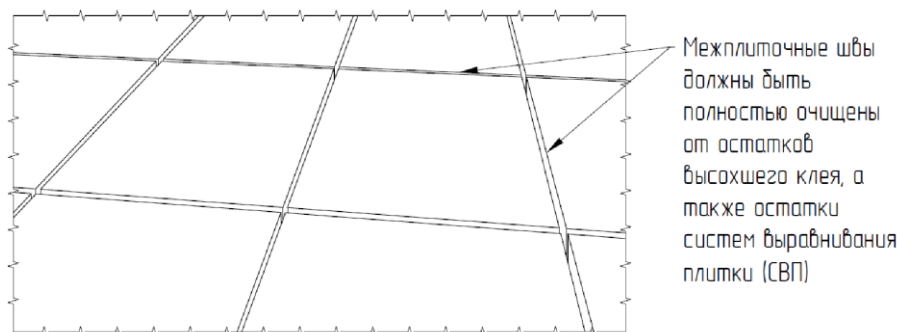
Рис. 38. Подготовка межплиточных швов
