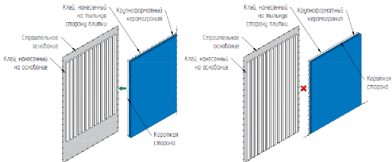
Рис. 32. Клей следует наносить в одном направлении на основание и на плитку
