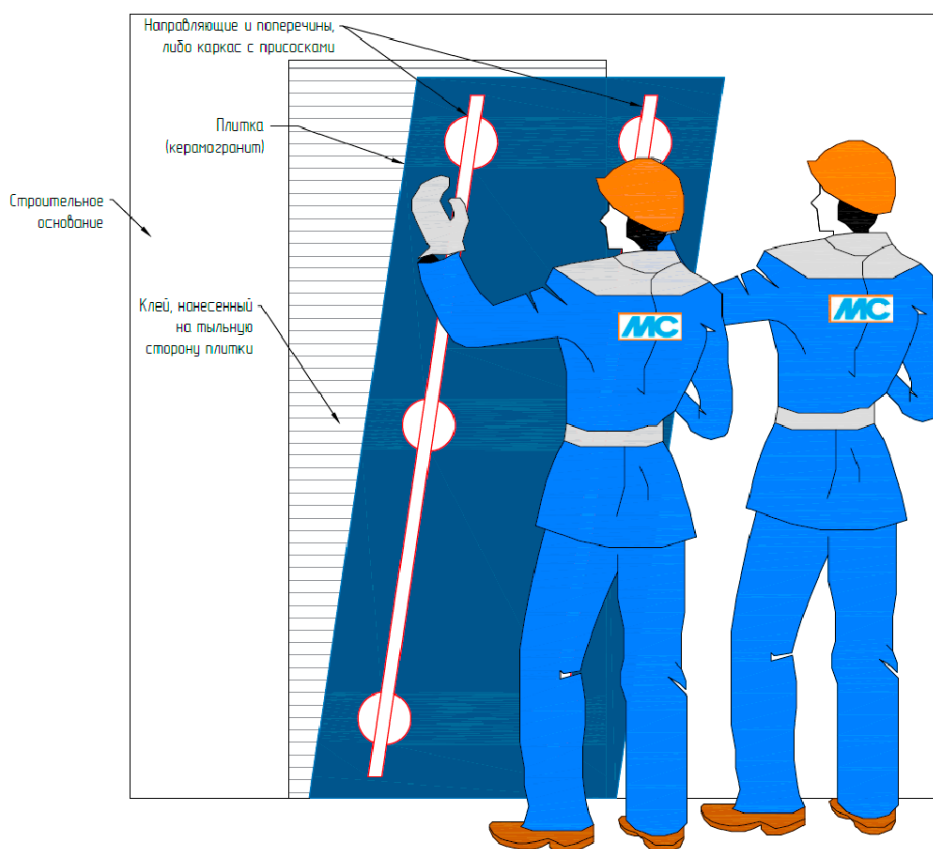
Рис. 35. Монтаж крупноформатного керамогранита
