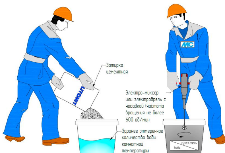
Рис. 39. Приготовление состава
