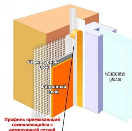
Рис.12. Профиль примыкающий с армирующей сеткой
