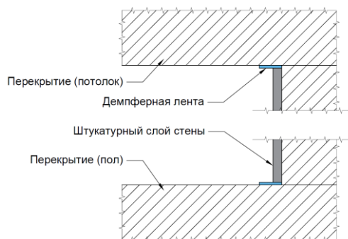
Рис.11. Приклейка демпферной ленты в местах сопряжения штукатурного слоя со стеной и потолком
