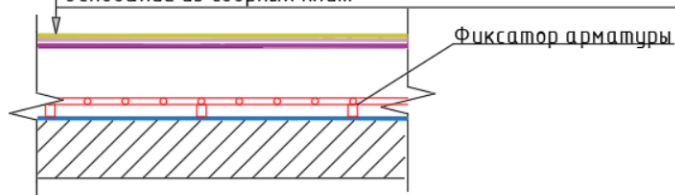
Сечение готового покрытия.
