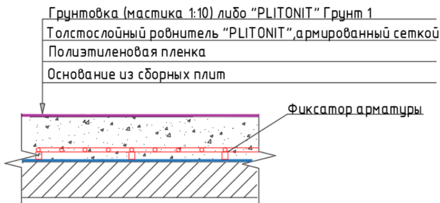
Сечение готового огрунтованного покрытия.
