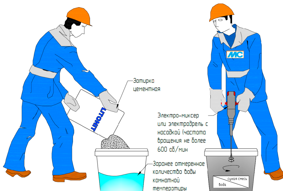
Рис. 11. Приготовление состава
