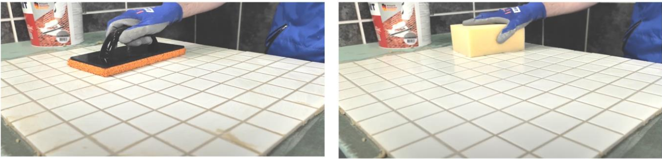
Рис. 14. Диагональными движениями шпателя убрать с поверхности плитки излишки затирки
