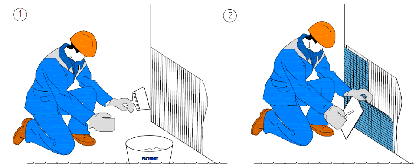
Рис. 9. Организация работ по приклеиванию мозаики
