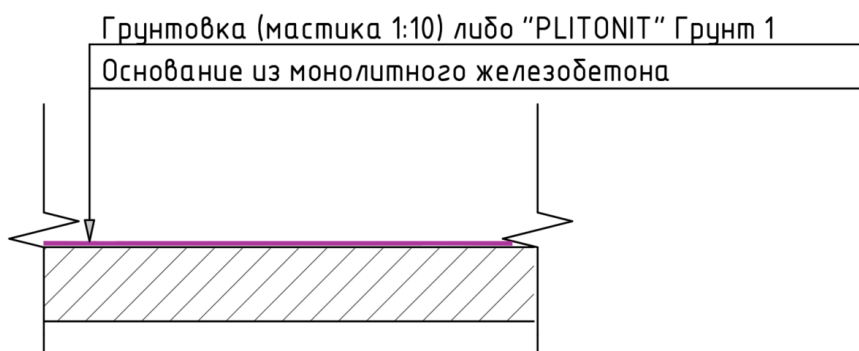
Сечение готового огрунтованного покрытия.
