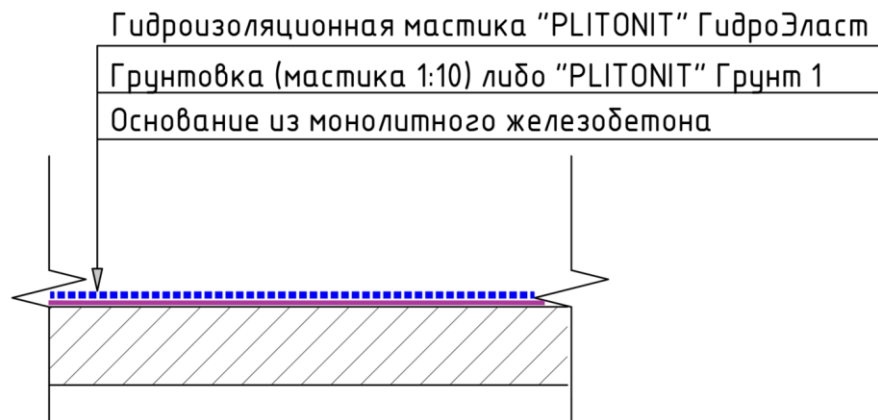
Сечение готового покрытия гидроизоляции.
