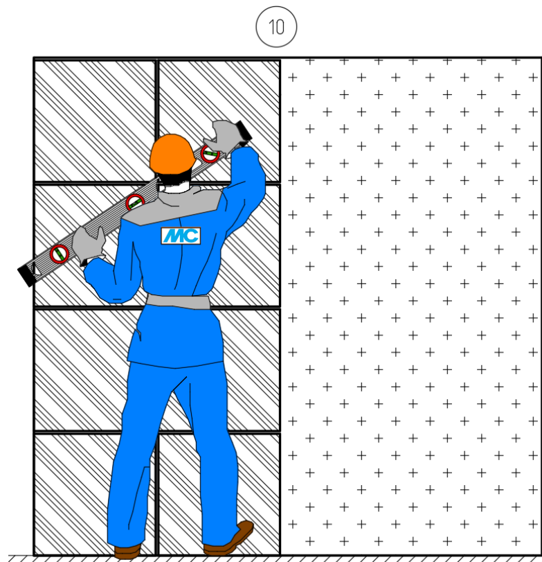
Рис.33. Последовательность работ, где: 1 – проверка ровности основания контрольной рейкой; 2, 3 – приготовление грунтовки; 4 – нанесение грунтовки на цементную штукатурку; 5 – приготовление клеевой смеси; 6, 7 – нанесение клеевой смеси на основание (захватками); 8, 9 – приклеивание керамогранитной плитки на стену (захватками); 10 – проверка облицовки при помощи уровня.
