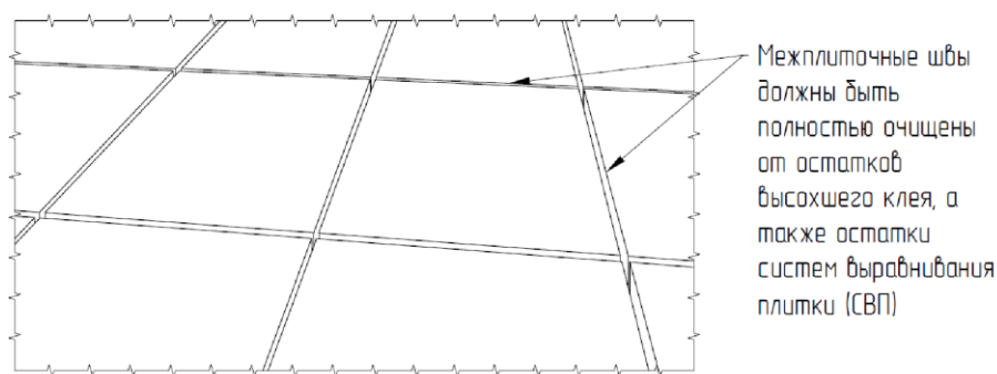
Рис. 34. Подготовка межплиточных швов
