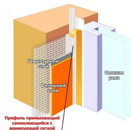
Рис.26. Профиль примыкающий с армирующей сеткой
