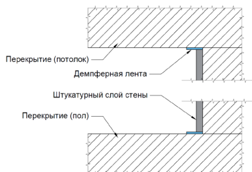
Рис.25. Приклейка демпферной ленты в местах сопряжения штукатурного слоя со стеной и потолком
