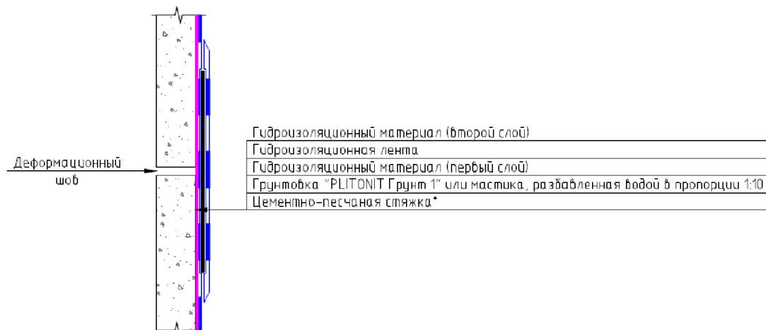
Рис.22.3. Конструктивный разрез №3.
