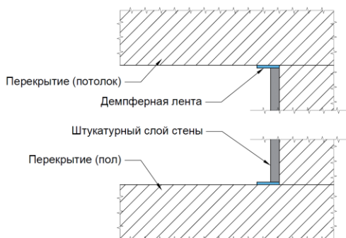
Рис.27. Приклейка демпферной ленты в местах сопряжения штукатурного слоя со стеной и потолком
