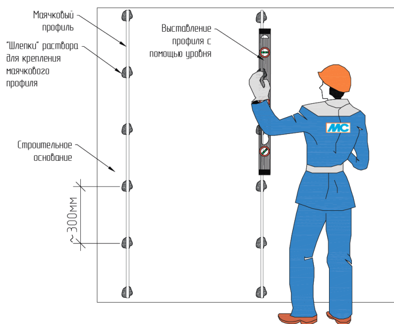
Рис.25. Монтаж маяка с помощью правила с уровнем
