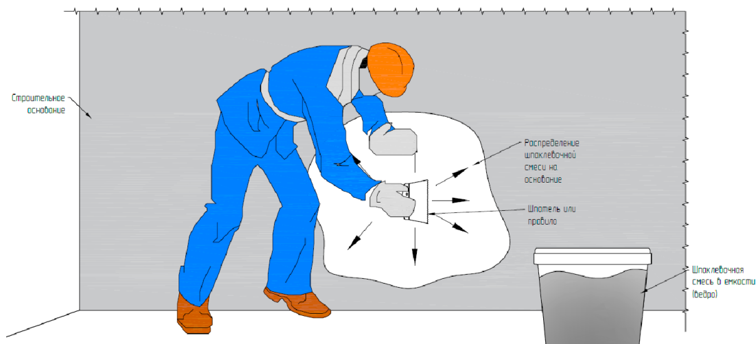
Рис. 25. Организация работ по нанесению шпаклевочной смеси
