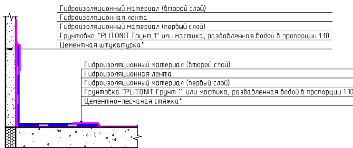
Разрез 1-1
