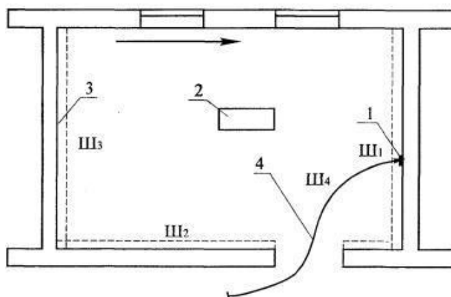
Рис. 21. Схема организации рабочего места звена № 1
