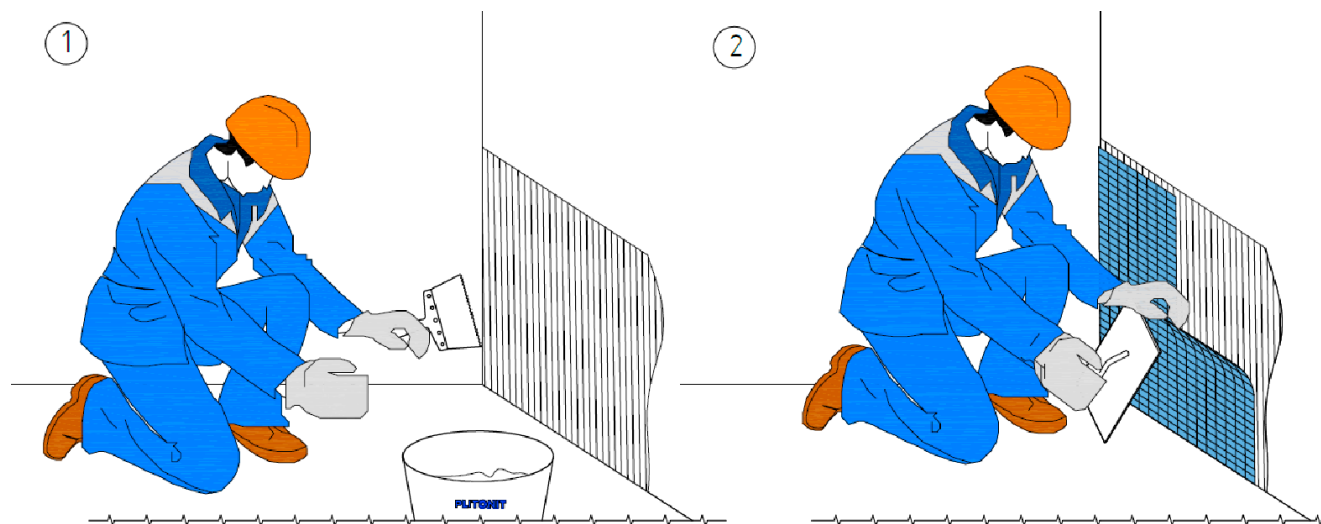
Рис. 29. Организация работ по приклеиванию мозаики
