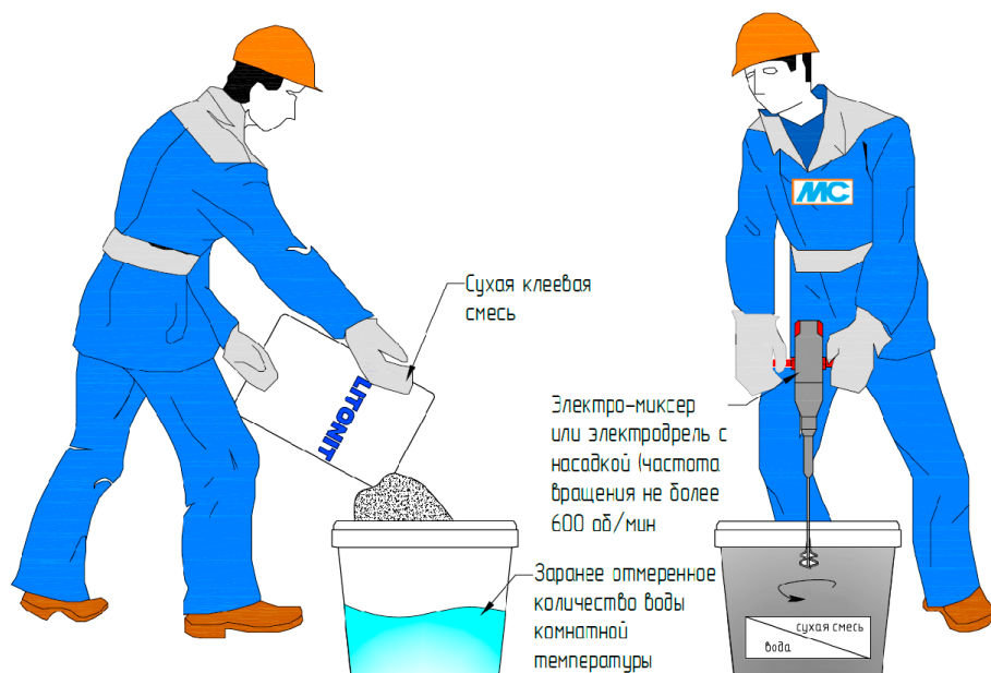
Рис. 28. Организация работ по затворению сухой клеевой смеси
