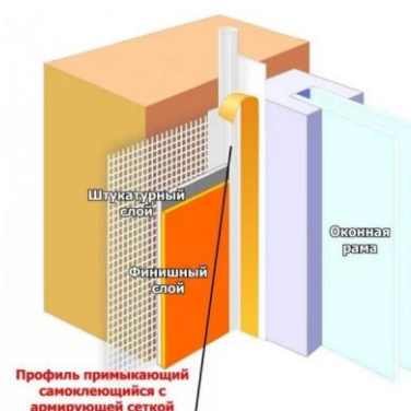
Рис.20. Профиль примыкающий с армирующей сеткой
