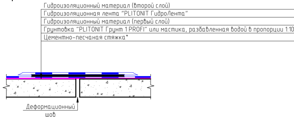
Рис.34. Конструктивный разрез №6.
