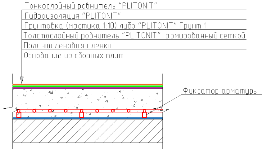
Рис.36. Конструктивный разрез №7.
