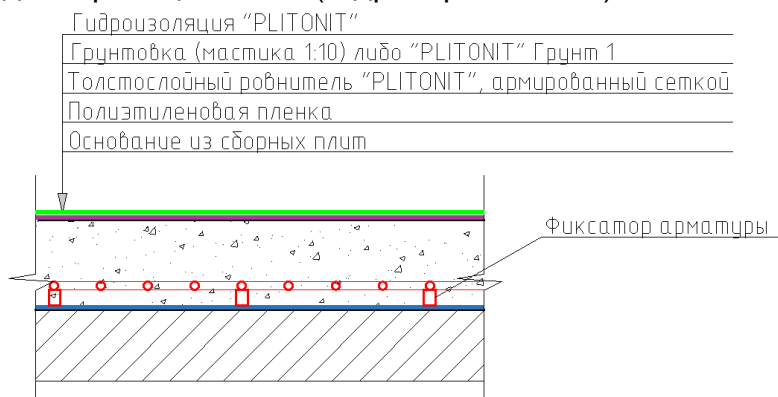
Рис.30. Конструктивный разрез №3
