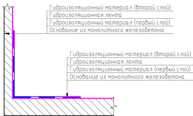
Рис.31. Устройство гидроизоляции внутренних углов с применением «PLITONIT ГидроЛента» и «PLITONIT ГидроЛента угол внутренний 90°».
