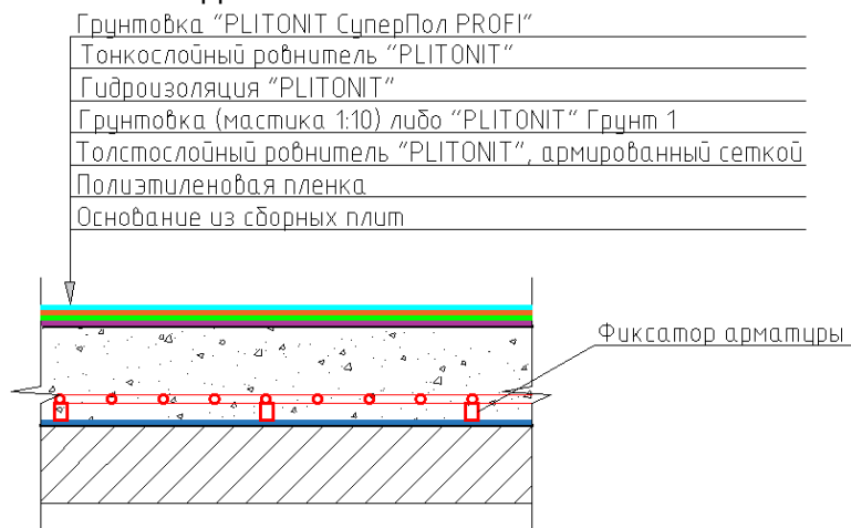
Рис.37. Конструктивный разрез №8.
