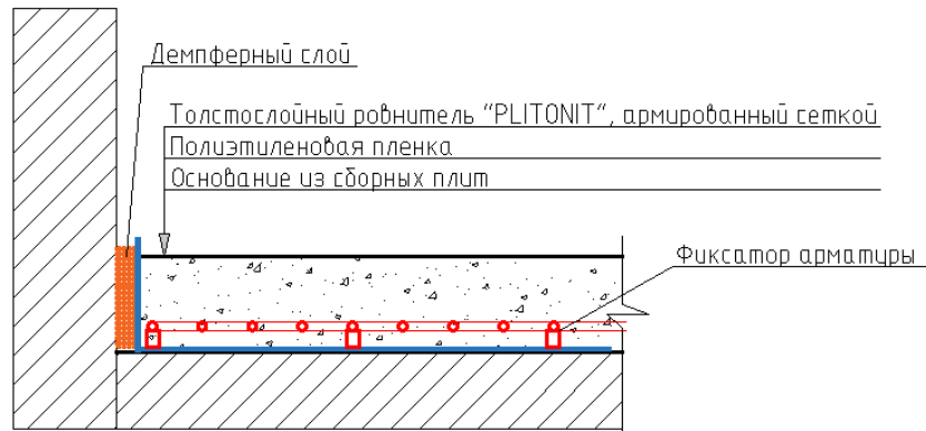
Рис.28. Конструктивный разрез №1.
