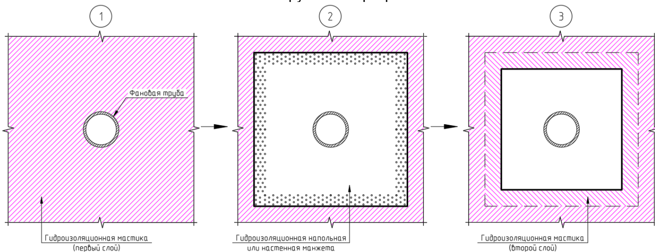
Рис.35. Последовательность нанесения гидроизоляционной манжеты.
