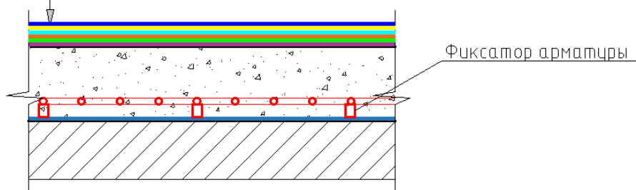
Рис.38. Конструктивный разрез №9.
