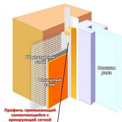
Рис.23. Профиль примыкающий с армирующей сеткой
