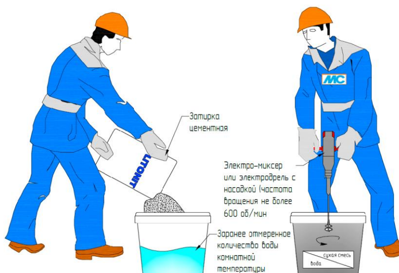
Рис. 39. Приготовление состава
