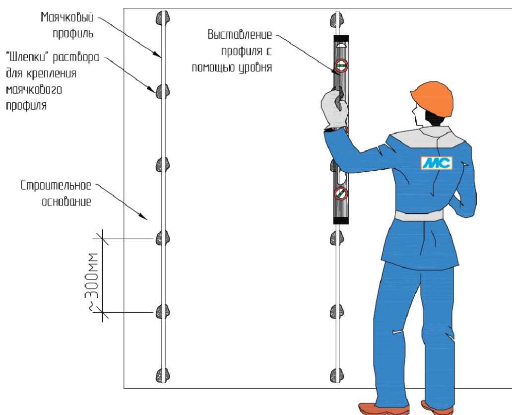
Рис.18. Монтаж маяка с помощью правила с уровнем
