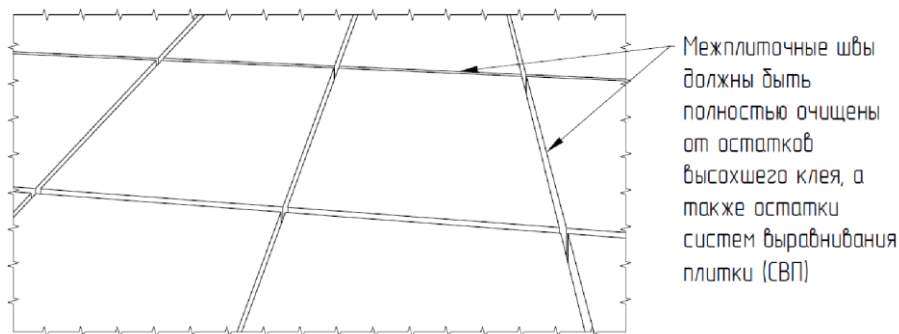
Рис. 32. Подготовка межплиточных швов
