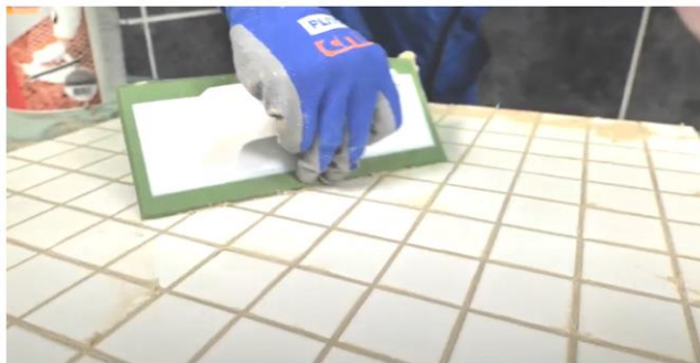
Рис. 35. Диагональными движениями шпателя убрать с поверхности плитки излишки затирки
