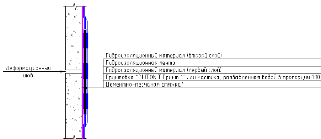
Рис.25.3. Конструктивный разрез №3.
