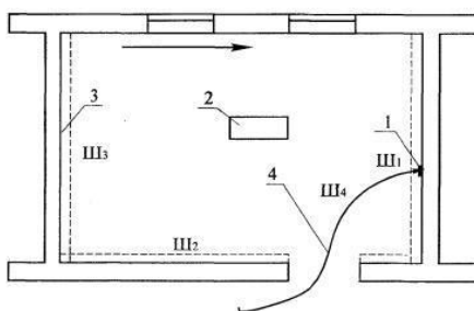
Рис. 21. Схема организации рабочего места звена № 1
