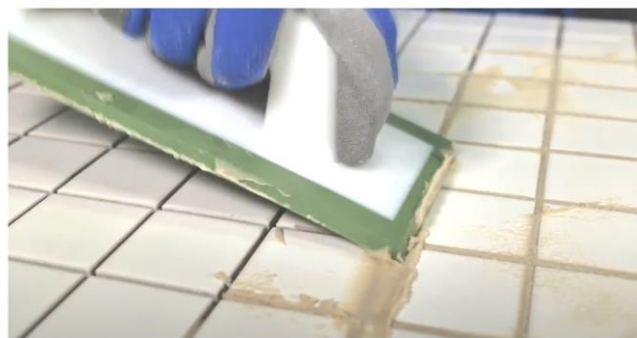
Рис. 31. Заполнение швов затиркой при помощи резинового шпателя
