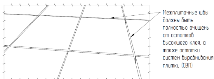
Рис. 29. Подготовка межплиточных швов
