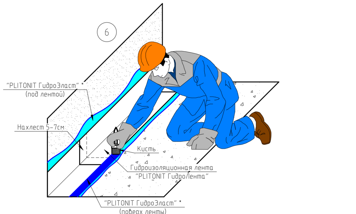
Рис.26.1. Последовательность работ (на стенах работа в аналогичном порядке), где: 1 - проверка ровности основания контрольной рейкой (аналогично для горизонтальной поверхности); 2 – размешивание емкости с мастикой; 3 – нанесение первого слоя мастики, разбавленной водой в пропорции 1:10, на основание; 4 – нанесение гидроизоляции на поверхность (аналогично для горизонтальной поверхности); 5 – укладка гидроизоляционной ленты на поверхность, предварительно обработанную «PLITONIT ГидроЭласт» или «PLITONIT WaterProof Standard»; 6 – поверхностная обработка ленты мастикой «PLITONIT ГидроЭласт» или «PLITONIT WaterProof Standard»
