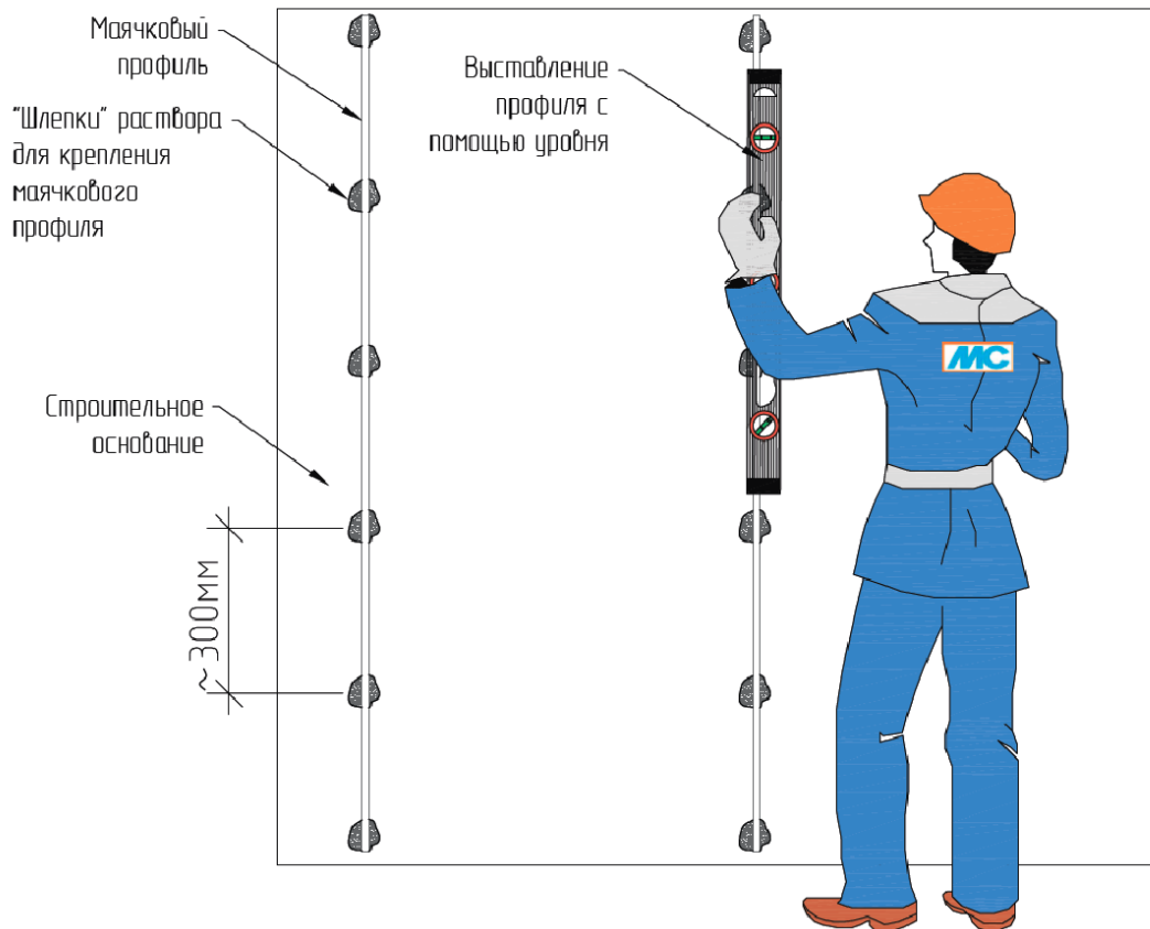
Рис.17. Монтаж маяка с помощью правила с уровнем
