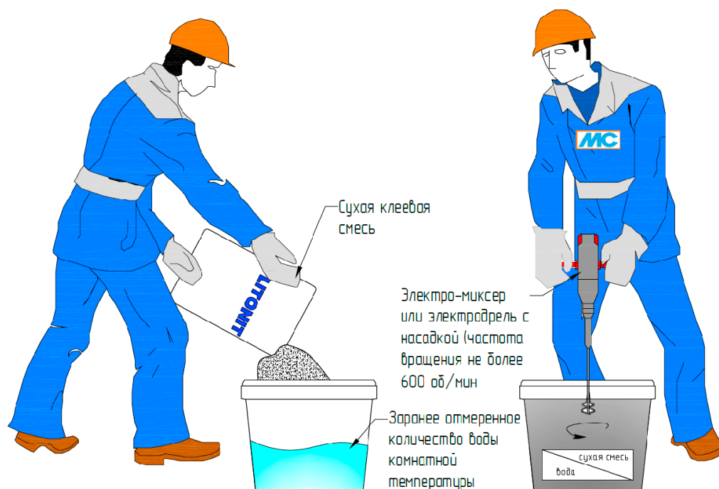
Рис. 27. Организация работ по затворению сухой клеевой смеси
