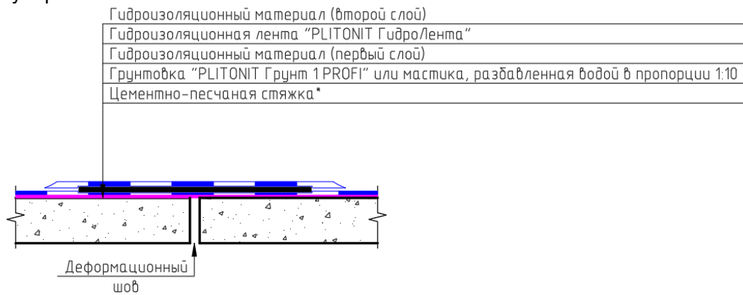
Рис.22. Конструктивный разрез №6.
