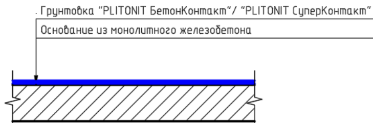
Рис.15. Конструктивный разрез №1.
