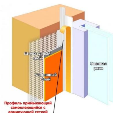
Рис.17. Профиль примыкающий с армирующей сеткой
