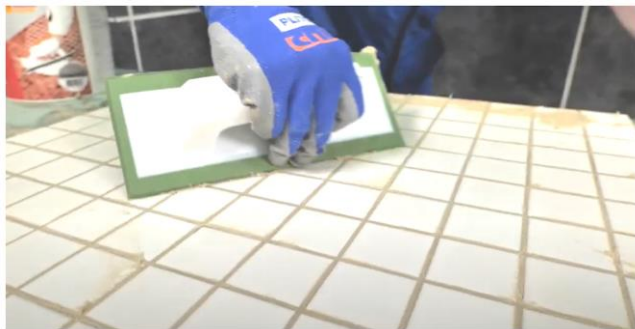
Рис. 30. Диагональными движениями шпателя убрать с поверхности плитки излишки затирки
