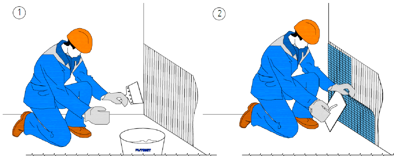
Рис. 26. Организация работ по приклеиванию мозаики
