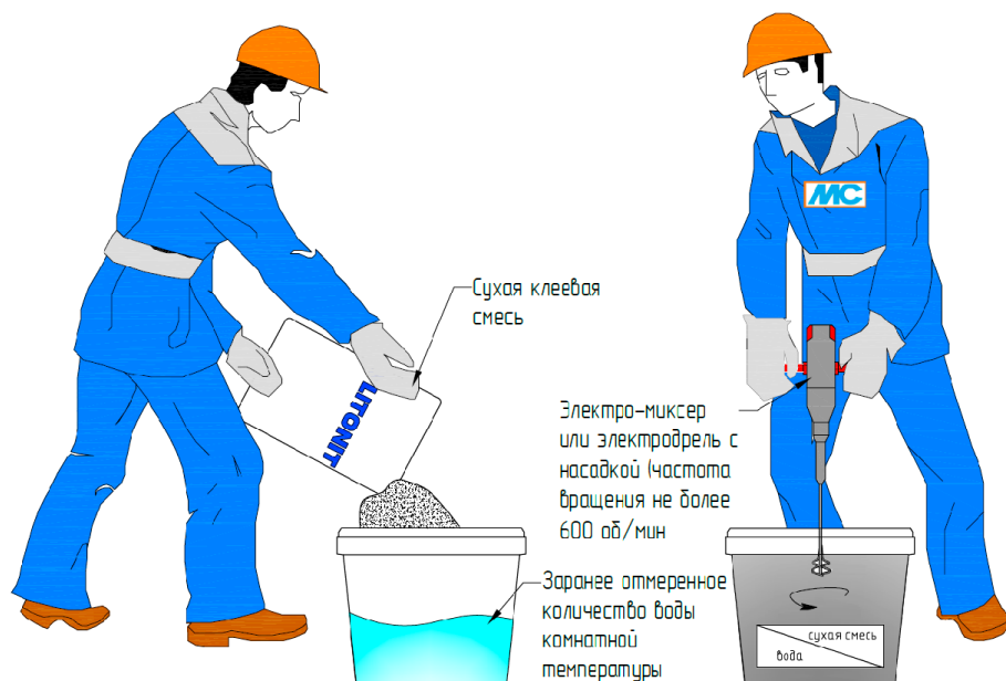
Рис. 31. Организация работ по затворению сухой клеевой смеси
