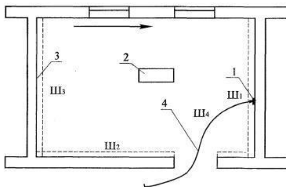
Рис. 23. Схема организации рабочего места звена № 1
