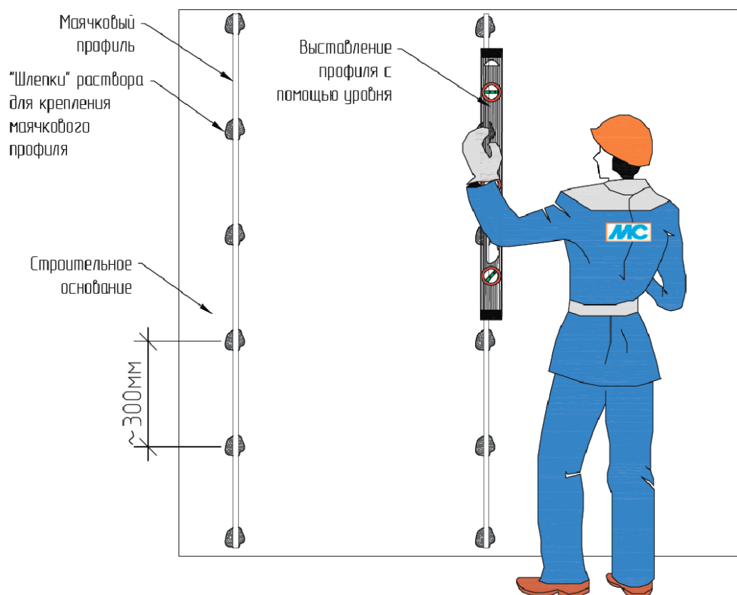
Рис.19. Монтаж маяка с помощью правила с уровнем
