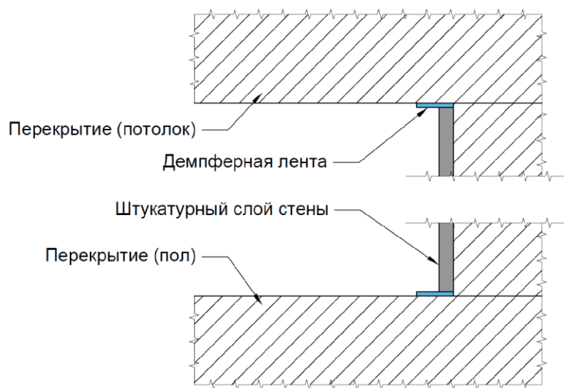
Рис.21. Приклейка демпферной ленты в местах сопряжения штукатурного слоя со стеной и потолком
