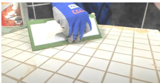
Рис. 36. Диагональными движениями шпателя убрать с поверхности плитки излишки затирки
