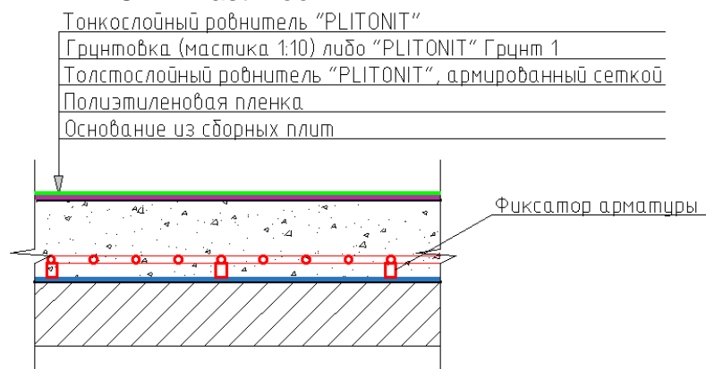
Рис.22. Конструктивный разрез №3.
