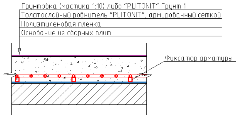
Рис.21. Конструктивный разрез №2.
