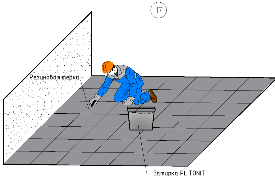
Рис.28. Последовательность работ, где: 1 – подготовка покрытия к укладке толстослойного ровнителя PLITONIT; 2 – приготовление смеси толстослойного ровнителя PLITONIT; 3-4– укладка толстослойного ровнителя PLITONIT; 5 – готовое покрытие толстослойного ровнителя PLITONIT; 6 – перемешка грунтовки PLITONIT; 7 – нанесение грунтовки PLITONIT; 8 – подготовка покрытия к укладке тонкослойного ровнителя PLITONIT; 9 – приготовление смеси тонкослойного ровнителя PLITONIT; 10– укладка тонкослойного ровнителя PLITONIT; 11 – готовое покрытие тонкослойного ровнителя PLITONIT; 12 – расправка грунтовки PLITONIT; 13 – перемешка грунтовки PLITONIT; 14 – нанесение грунтовки PLITONIT; 15 – нанесение клея PLITONIT; 16 – укладка плитки на клей PLITONIT; 17– затирка швов плитки составом PLITONIT.
