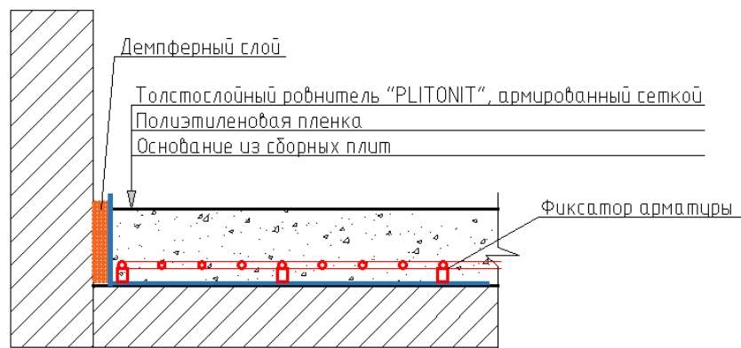
Рис.20. Конструктивный разрез №1.
