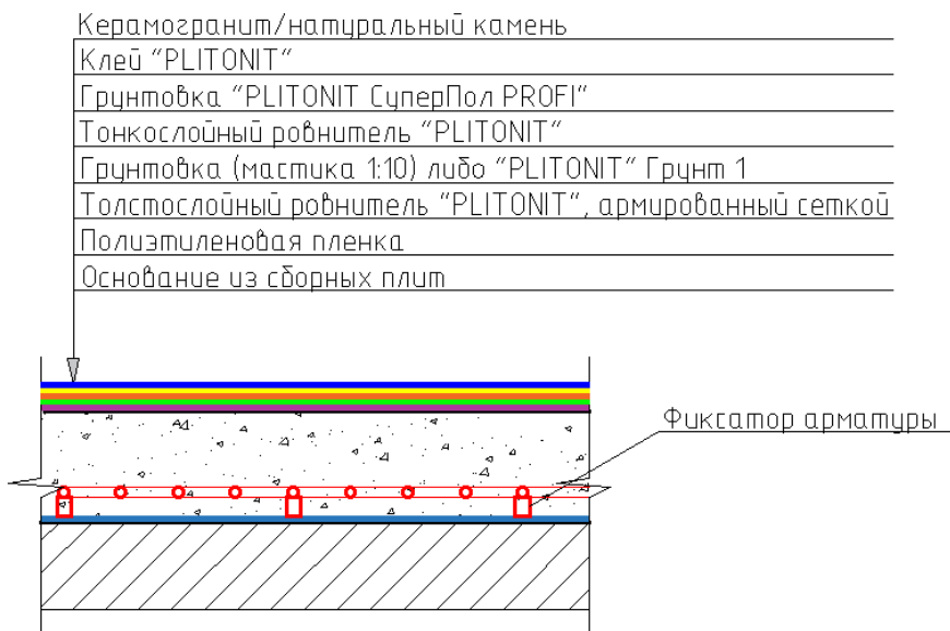
Рис.24. Конструктивный разрез №5.
