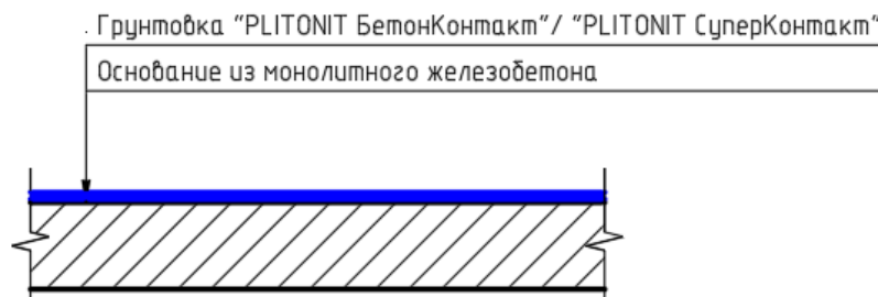
Рис.8. Конструктивный разрез №1.
