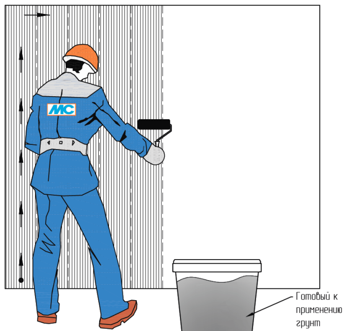
Рис. 19. Схема организации работ по нанесению грунта на основание
