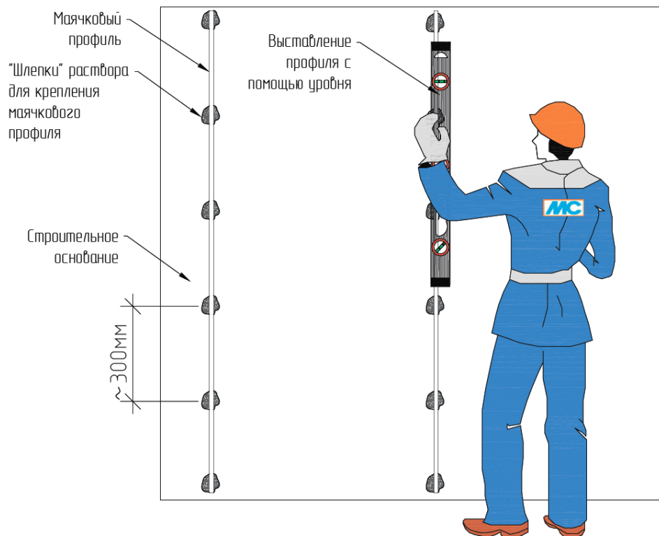
Рис.11. Монтаж маяка с помощью правила с уровнем
