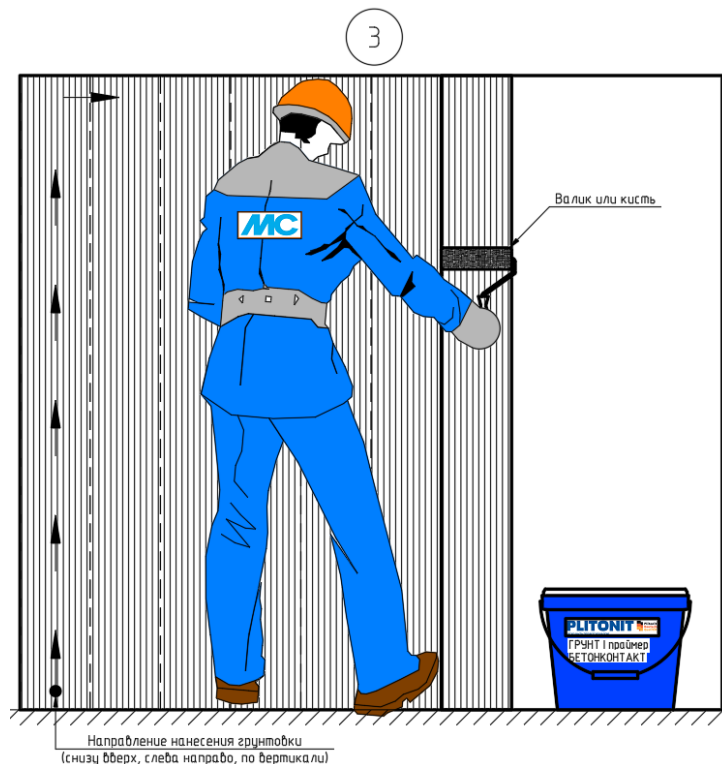
Рис.9. Последовательность работ.
