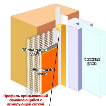
Рис.14. Профиль примыкающий с армирующей сеткой
