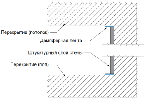
Рис.11. Приклейка демпферной ленты в местах сопряжения штукатурного слоя со стеной и потолком
