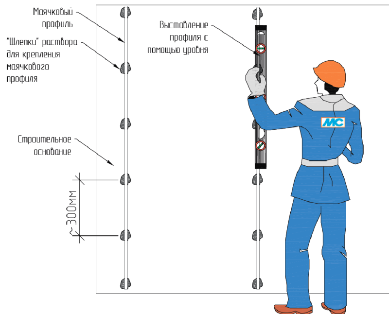
Рис.22. Монтаж маяка с помощью правила с уровнем
