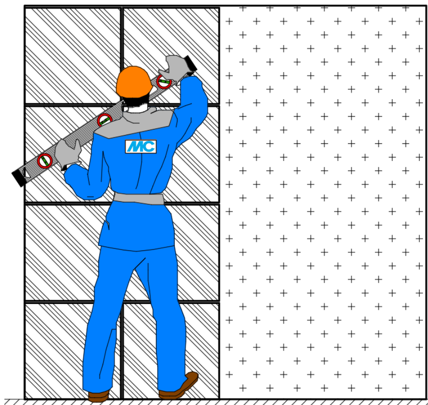
Рис.33. Последовательность работ, где: 1 – проверка ровности основания контрольной рейкой; 2, 3 – приготовление грунтовки; 4 – нанесение грунтовки на цементную штукатурку; 5 – приготовление клеевой смеси; 6, 7 – нанесение клеевой смеси на основание (захватками); 8, 9 – приклеивание керамогранитной плитки на стену (захватками); 10 – проверка облицовки при помощи уровня. ПРИМЕЧАНИЕ к рис 33.: на этапах 6-9 указано проведение работ в направлении снизу вверх, но при использовании клеев, в маркировке которых присутствует буква «Т», возможно выполнение работ в направлении сверху вниз.
