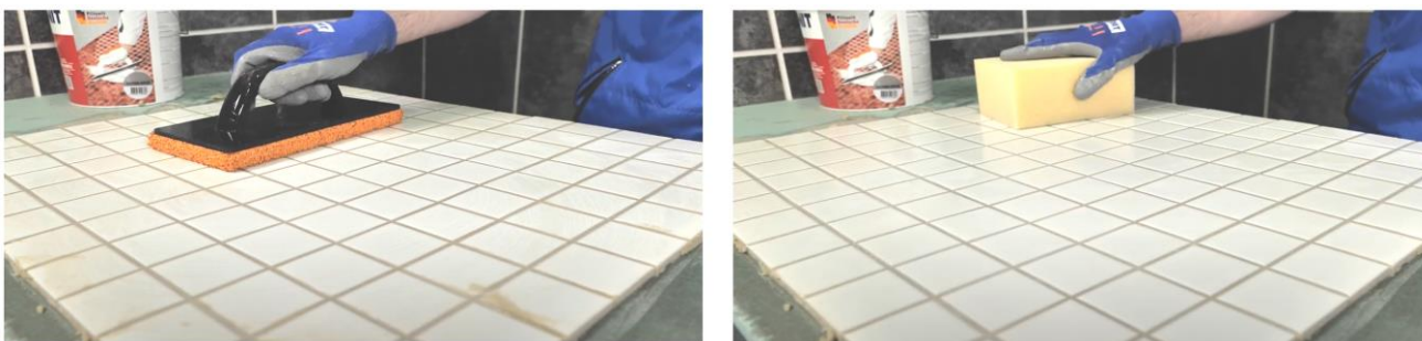
Рис. 38. Диагональными движениями шпателя убрать с поверхности плитки излишки затирки
