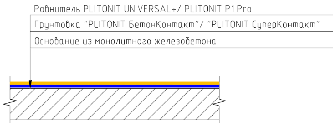
Рис.14. Конструктивный разрез №2.
