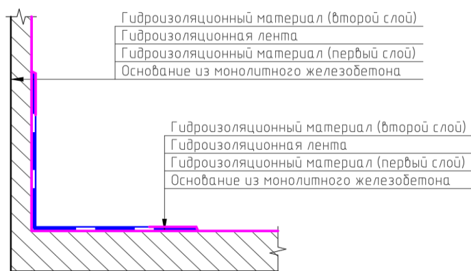
Рис.17. Устройство гидроизоляции внутренних углов с применением «PLITONIT ГидроЛента» и «PLITONIT ГидроЛента угол внутренний 90°».
