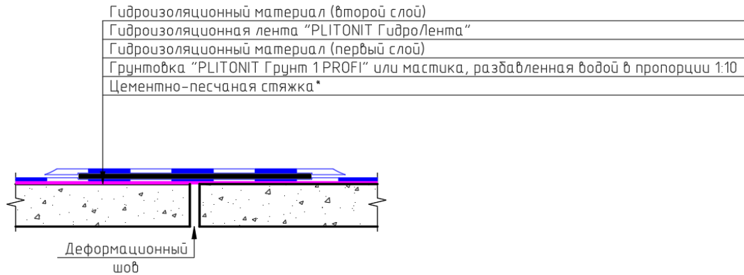
Рис.20. Конструктивный разрез №6.
