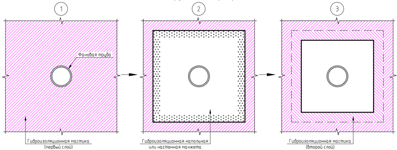
Рис.21. Последовательность нанесения гидроизоляционной манжеты.
