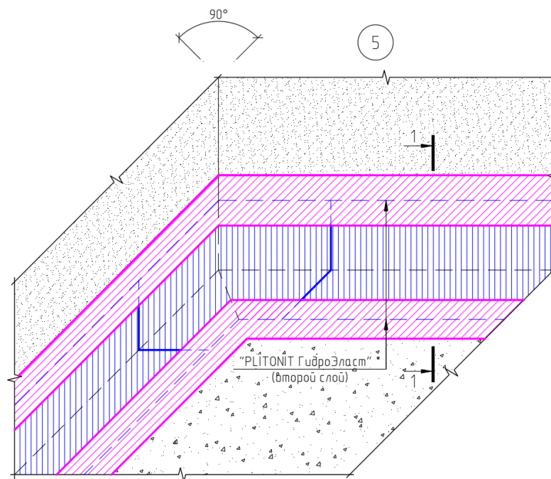
Разрез 1-1
