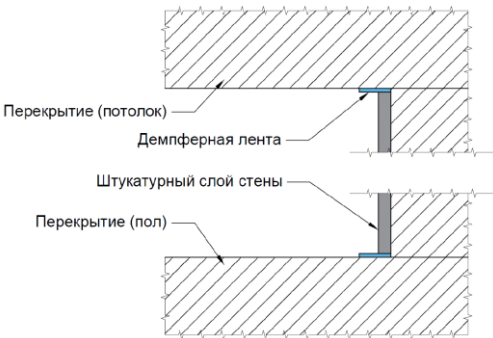
Рис.9.2. Приклейка демпферной ленты в местах сопряжения штукатурного слоя со стеной и потолком Для формирования примыкания штукатурки к листу ГКЛ (возможное применение: оконные откосы) используется штукатурный уголок (см. Рис. 10).
