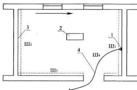
Рис. 11. Схема организации рабочего места звена № 1
