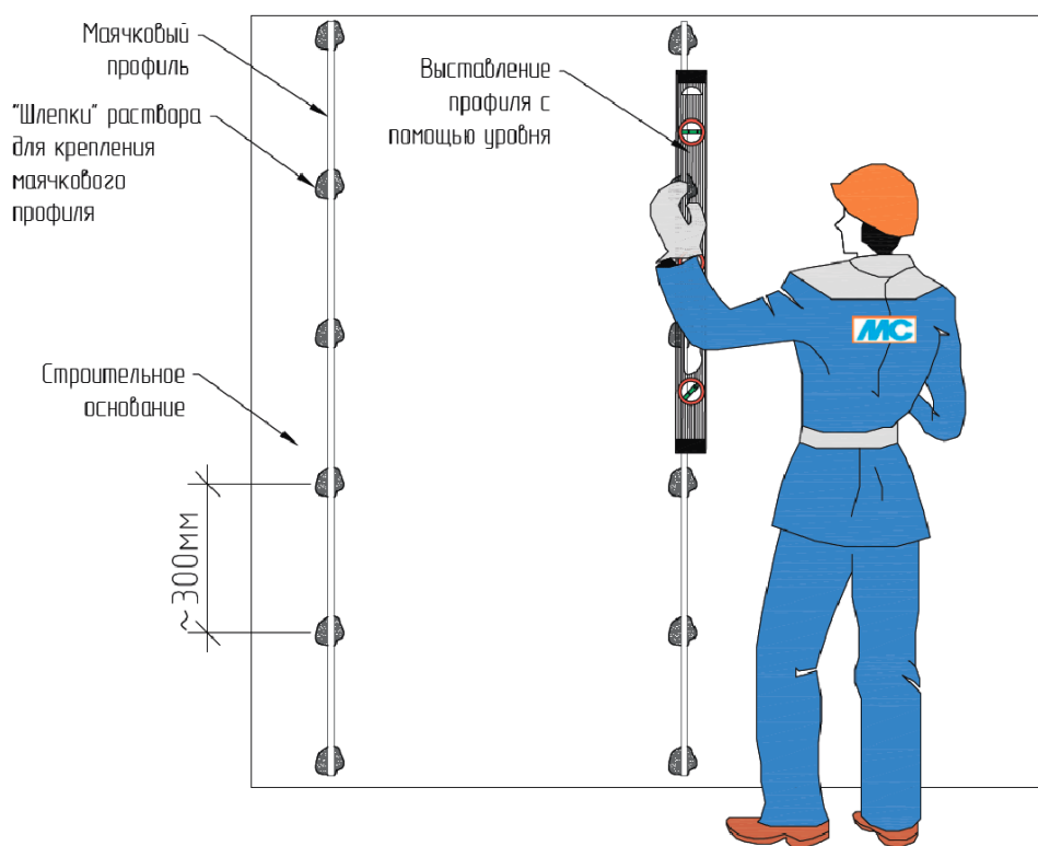
Рис.7. Монтаж маяка с помощью правила с уровнем
