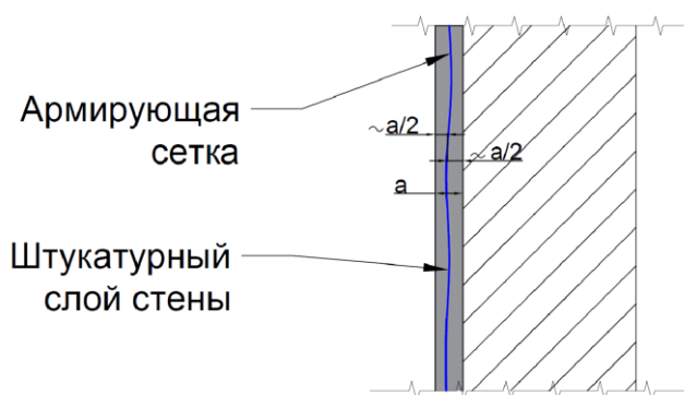
Рис. 13. Армированный штукатурный слой в местах стыка разных материалов стен
