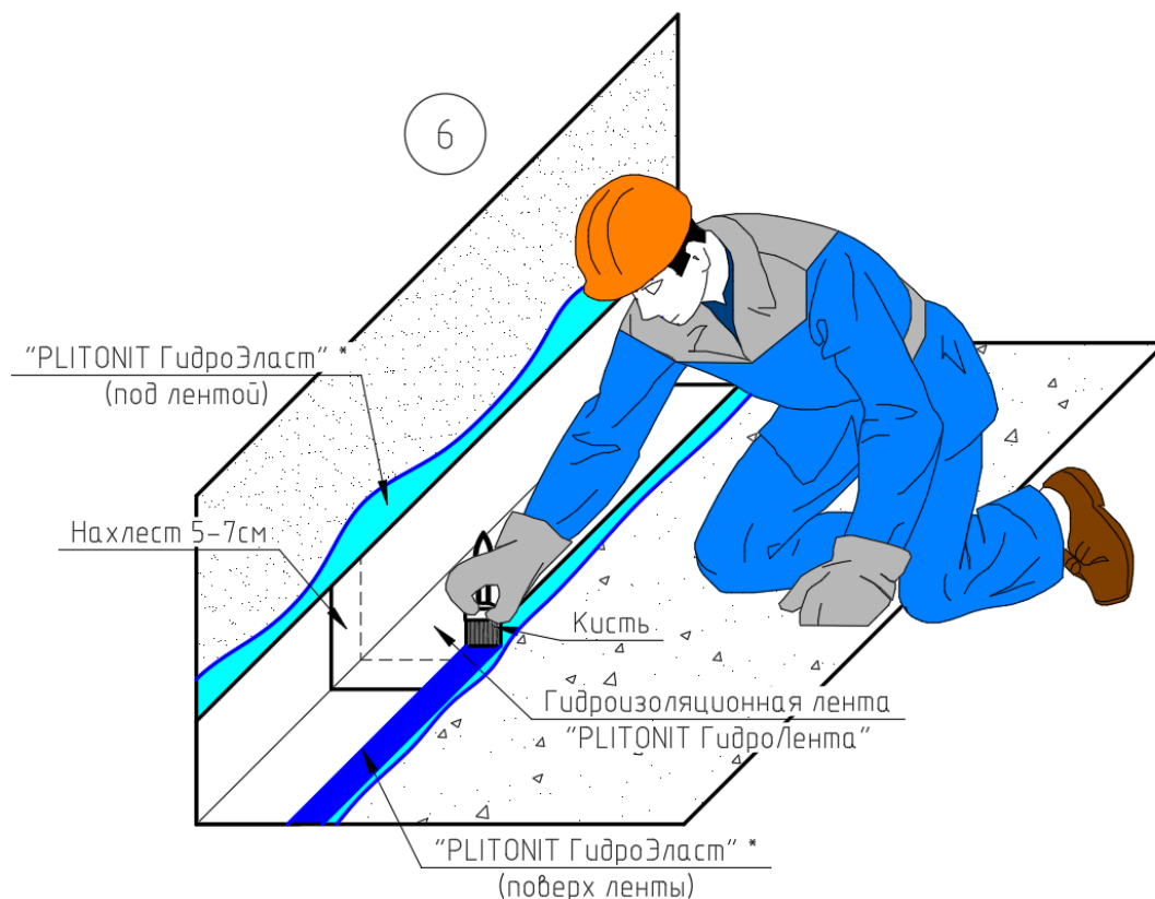
Рис.12. Последовательность работ, где: 1 - проверка ровности основания контрольной рейкой (аналогично для горизонтальной поверхности); 2 – размешивание емкости с мастикой; 3 – нанесение первого слоя мастики, разбавленной водой в пропорции 1:10, на основание; 4 – нанесение гидроизоляции на поверхность (аналогично для горизонтальной поверхности); 5 – укладка гидроизоляционной ленты на поверхность, предварительно обработанную «PLITONIT ГидроЭласт» или «PLITONIT WaterProof Standard»; 6 – поверхностная обработка ленты мастикой «PLITONIT ГидроЭласт» или «PLITONIT WaterProof Standard».
