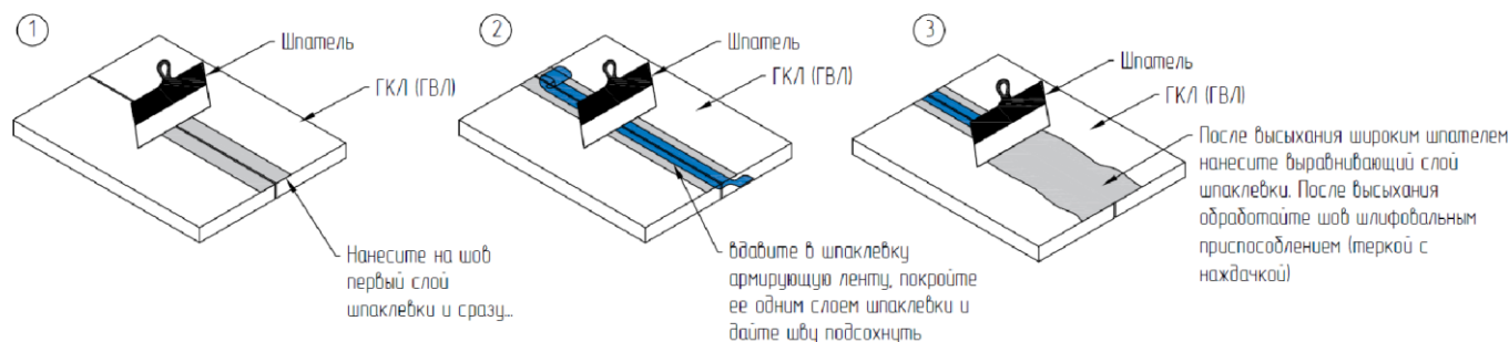
Рис. 15. Порядок шпаклевки швов между листов ГКЛ (ГВЛ) с использованием армирующей сетки
